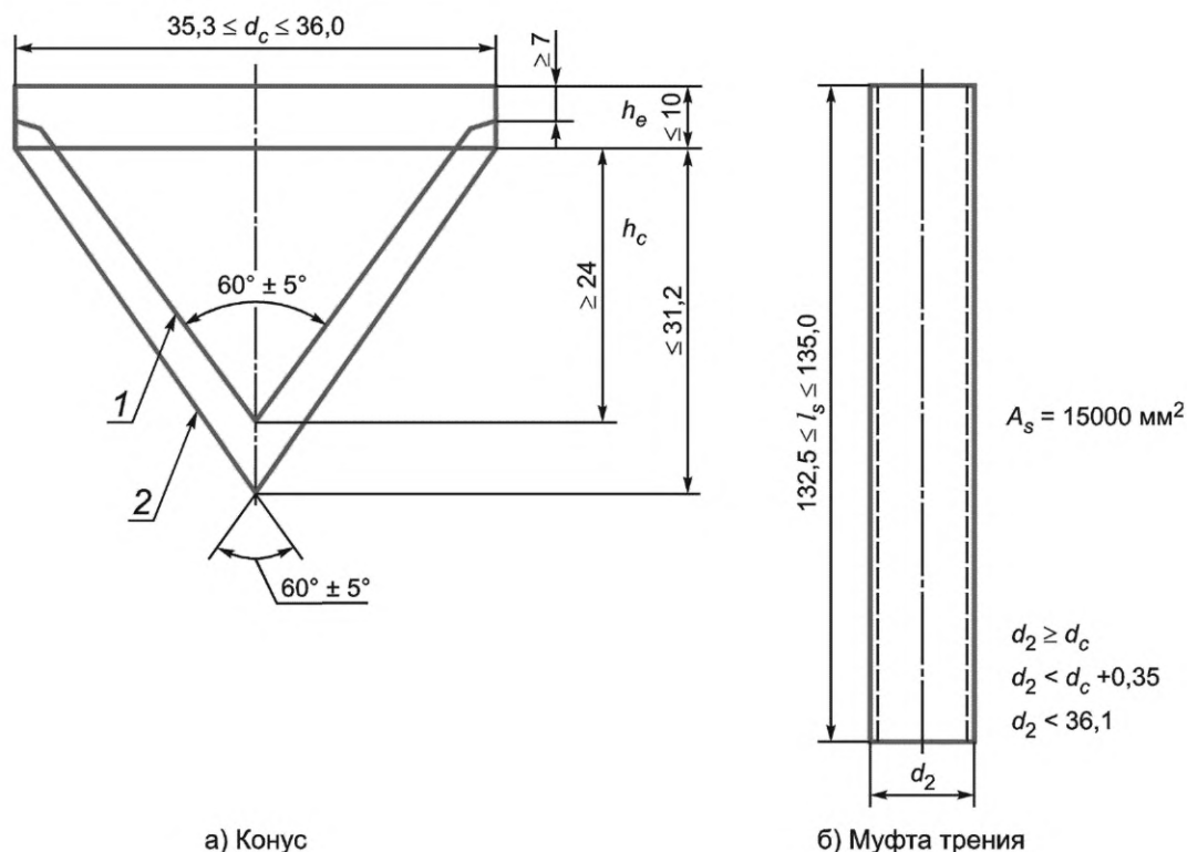
1 — минимальный размер изношенного конуса; 2 — максимальный размер конуса
