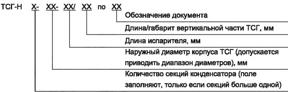
Рисунок 3 — Схема условного обозначения пологонаклонного ТSG
