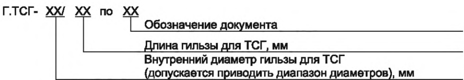
Рисунок 4 — Схема условного обозначения гильзы для ТSG
