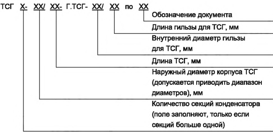
Рисунок 2 — Схема условного обозначения вертикального ТSG, устанавливаемого в гильзу для ТSG
