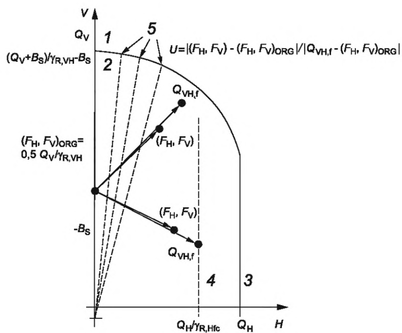
b) Глина с выталкивающей силой, действующей на башмак без засыпки на башмаке опоры
