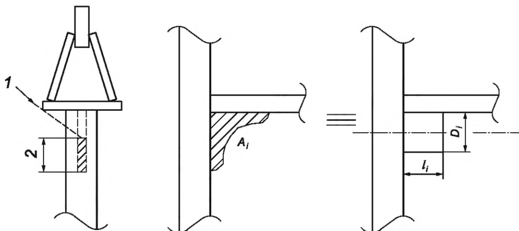
1 — направление потока; 2 — видимая часть углового соединения i ; A_i — площадь углового соединения i ; A_i = l_i D_i ; D_i — относительный диаметр углового соединения i ; l_i — относительная длина углового соединения i
