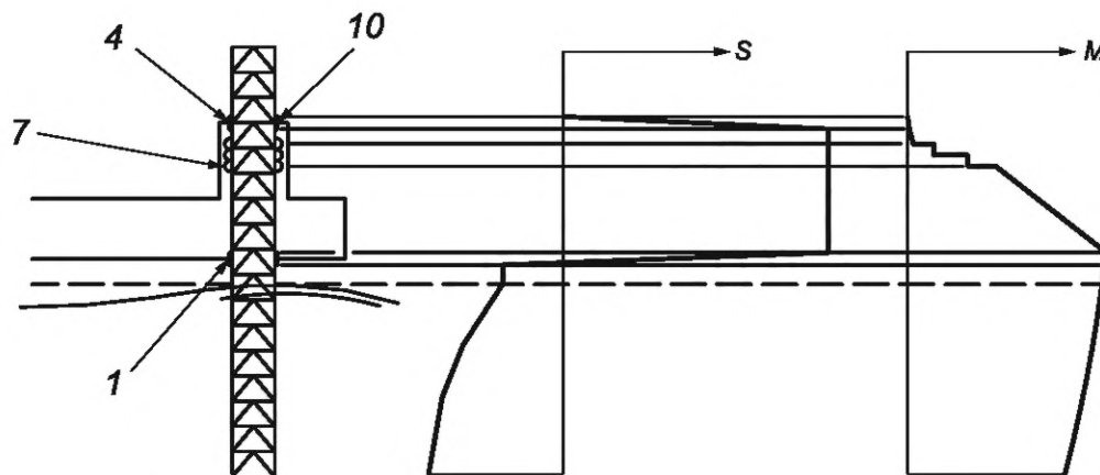
д) СПБУ без системы фиксации и имеющей плавающую подъемную систему
