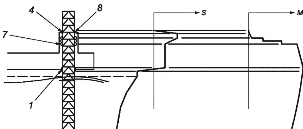
с) СПБУ без системы фиксации и имеющие неподвижную подъемную систему с непротивоположными шестернями
