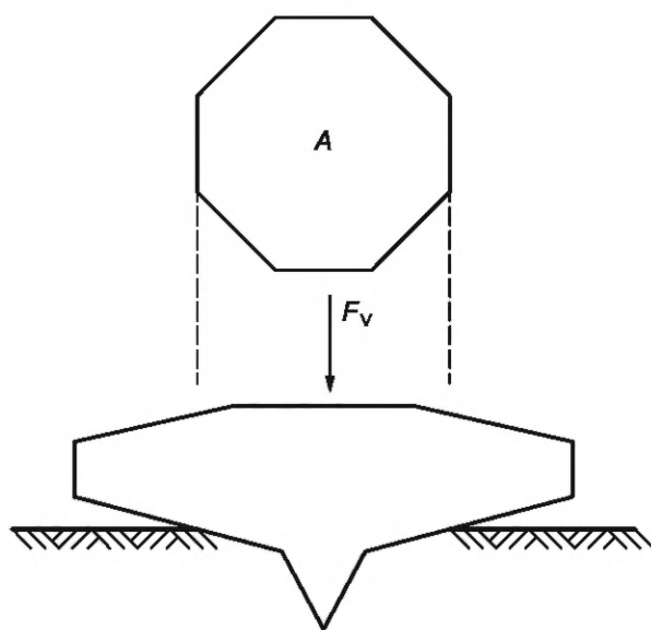
a) Реальный башмак опоры — частично погруженный
