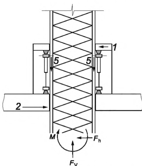
d) Подъемная система с фиксирующим стержнем и хомутом
