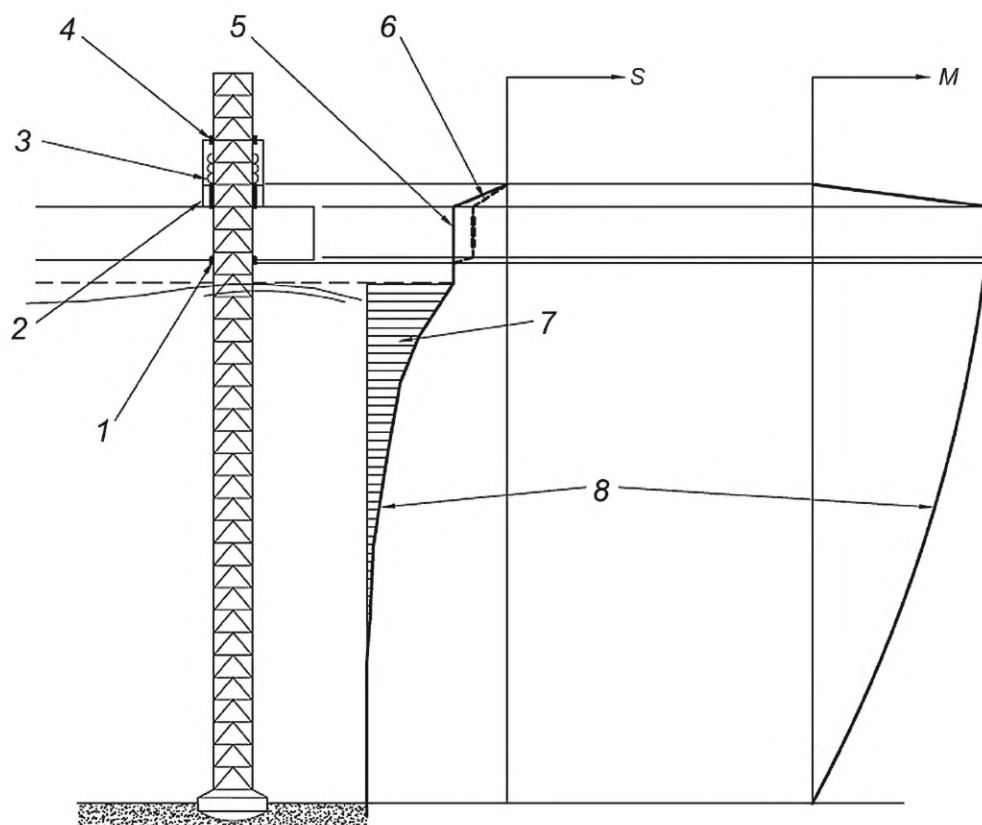
1 — нижняя направляющая; 2 — нижняя система фиксации; 3 — подъемная шестерня; 4 — верхняя направляющая; 5 — сдвигающая сила без контакта нижней направляющей; 6 — сдвигающая сила с контактом нижней направляющей; 7 — сдвиг из-за воздействия волн/течения; 8 — фактический сдвиг или изгибающий момент; S — сдвигающая сила; M — изгибающий момент
