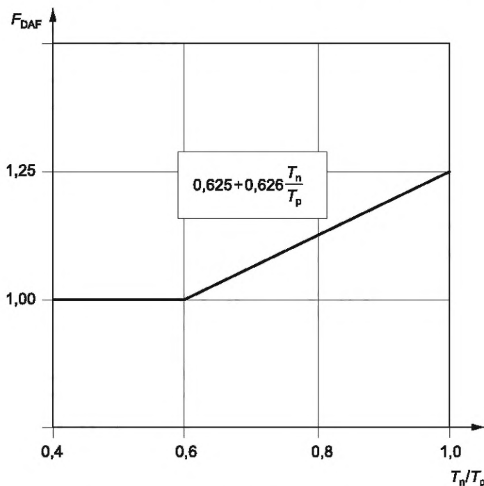
Рисунок С.3 — Графическое представление коэффициента масштабирования КДУ F_{KDU} , применяемое к методу инерции сопротивления
