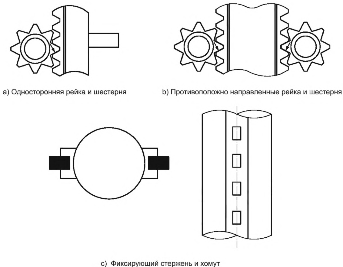
Рисунок А.8 — Типы подъемных систем
