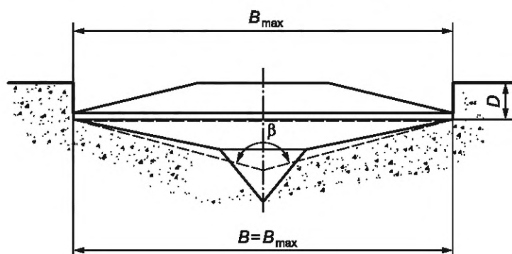
д) Полное прилегание ниже поверхности морского дна
