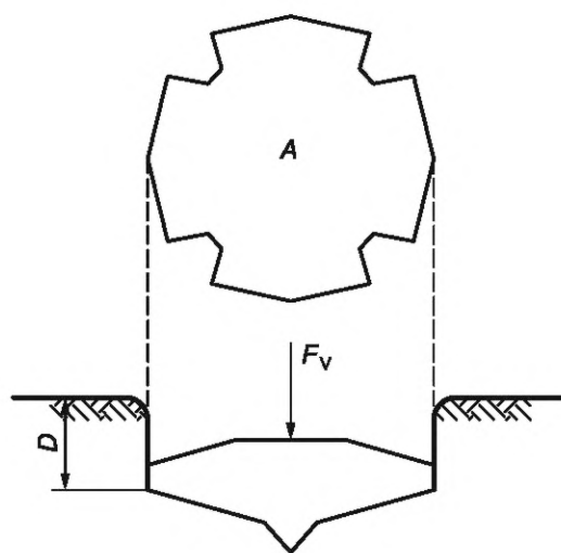
b) Реальный башмак опоры — полностью погруженный
