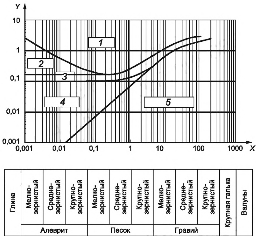
X — размер частиц в миллиметрах; Y — средняя скорость потока в метрах в секунду; 1 — эрозия; 2 — транспортирование/эрозия; 3 — транспортирование; 4 — седиментация/транспортирование; 5 — седиментация
