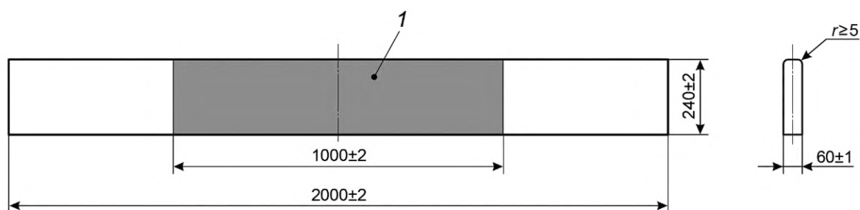
Рисунок 2 — Доска упора
