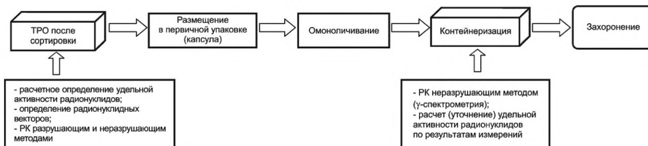
Рисунок Б.5 — Производственно-технологическая цепочка обращения с твердыми ВАО и САО, образовавшимися на АС в результате активации, с указанием этапов проведения РК
