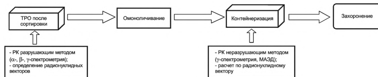
Рисунок Б.4 — Производственно-технологическая цепочка обращения с неперерабатываемыми РАО АС с указанием этапов проведения РК
