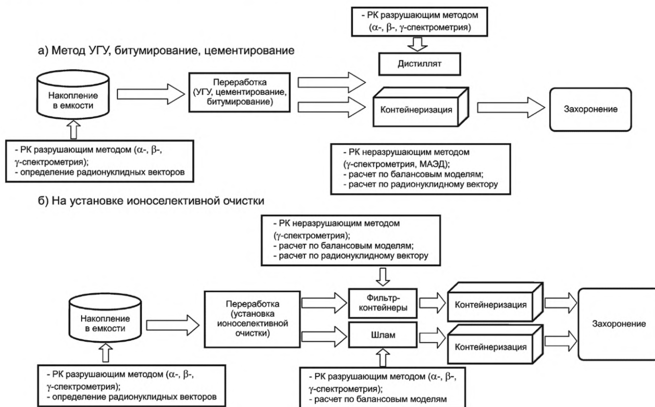
Рисунок Б.1 — Производственно-технологическая цепочка обращения с отверждаемыми ЖРО с указанием этапов проведения РК
