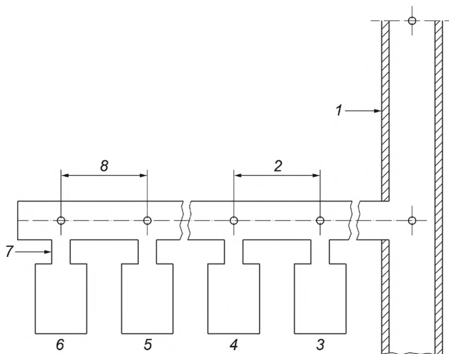
1 — конструкция для удаления дымовых газов; 2 — коллекторная секция j, l ; 3 — источник тепла j, l+1 ; 4 — источник тепла j, l ; 5 — источник тепла j, 2 ; 6 — источник тепла j, 1 ; 7 — соединительный элемент; 8 — коллекторная секция j, 1
