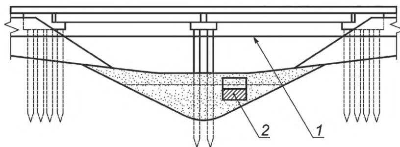
Рисунок 5 — Противоналедный мост-труба
