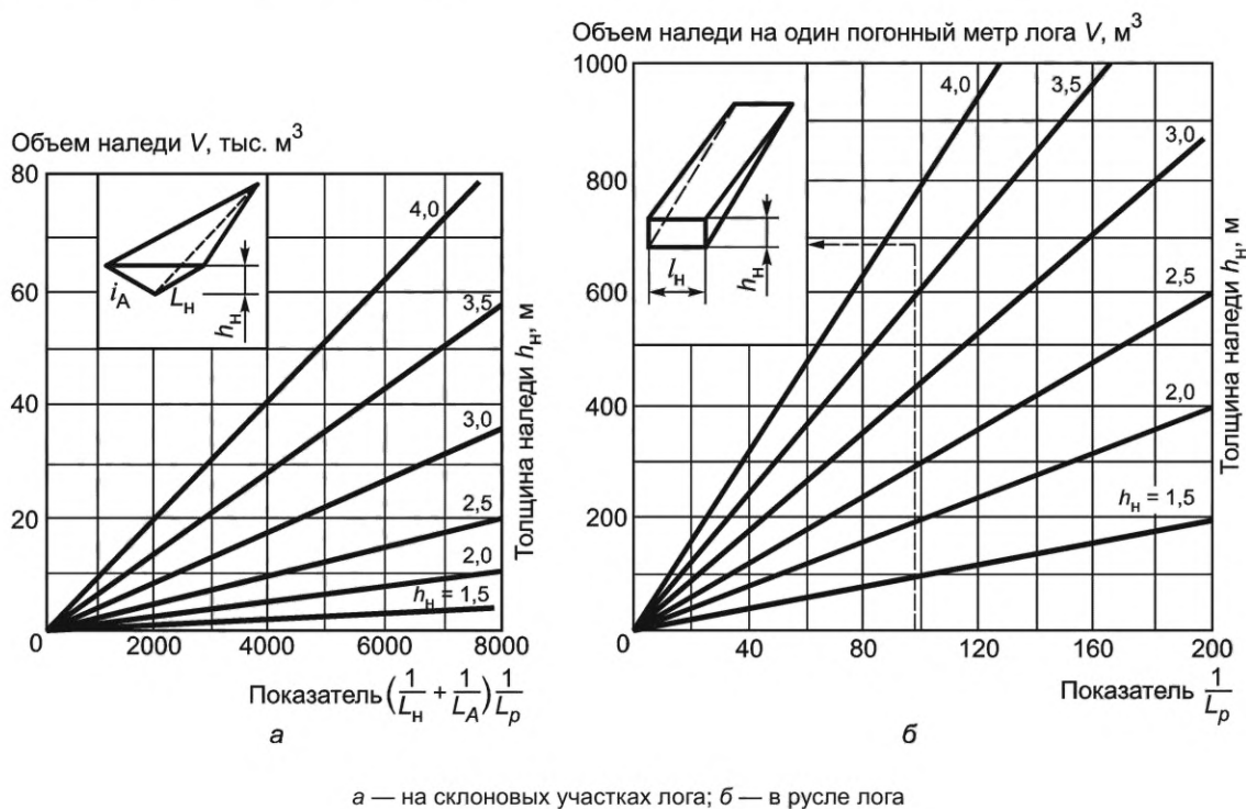
Рисунок Ж.2 — Графики зависимости объема наледи от ее толщины, формы поперечного сечения лога, уклонов главного русла и склонов
