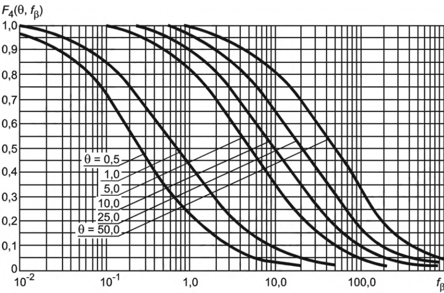
Рисунок В.8 — Графики функции F_4(\theta, f_\beta)
