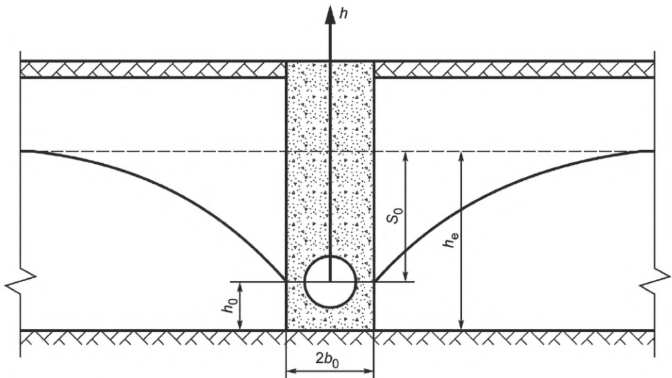
Рисунок В.1 — Схема к расчету однолинейного горизонтального дренажа совершенного типа
