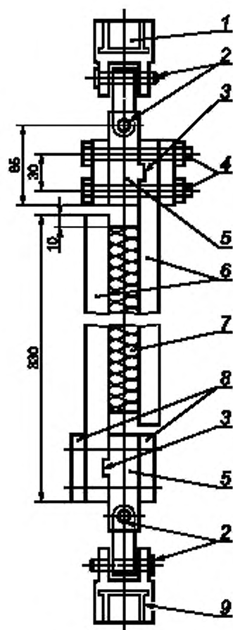
1 — неподвижный зажим испытательной машины; 2 — соединительные штифы универсального соединения; 3 — гребень и паз; 4 — крепление из гаек и болтов; 5 — адаптер; 6 — держатели для образца (длина 330, ширина 50, толщина 16 мм); 7 — образец (длина 250, ширина 50 мм); 8 — пластины распределения нагрузки; 9 — подвижный зажим испытательной машины
