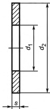
Рисунок 1 – Конструкция увеличенной шайбы
