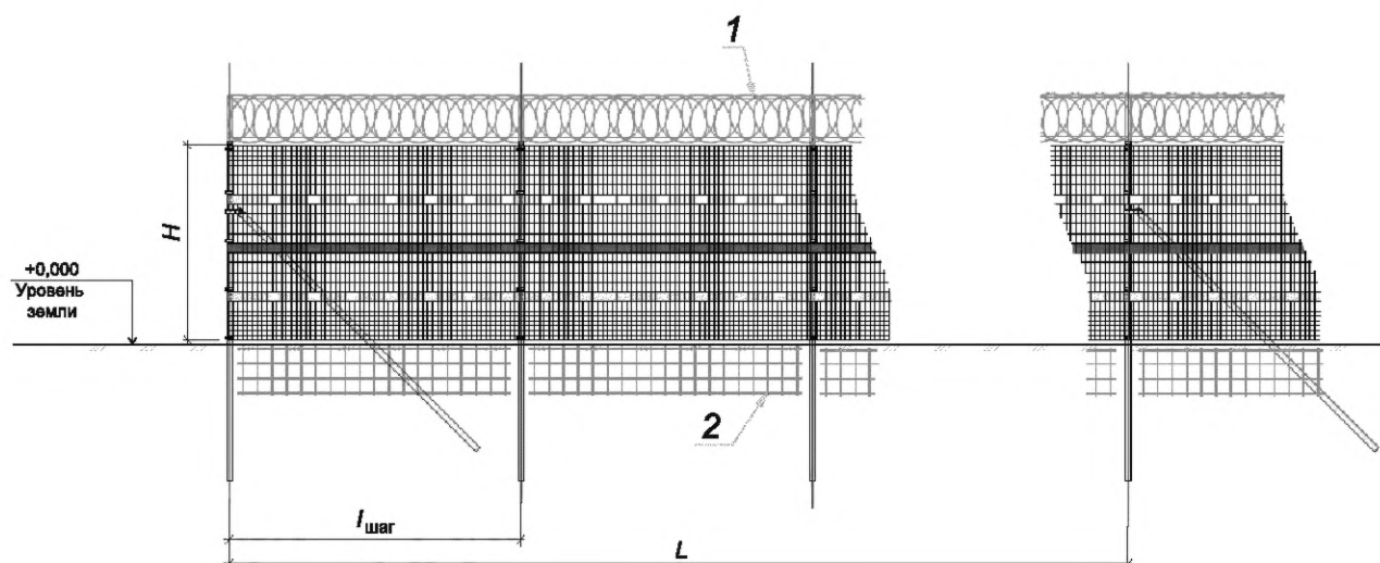
1 — дополнительное ограждение; 2 — противоподкопное усиление
