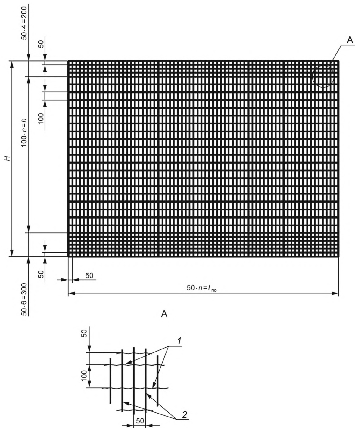
Рисунок 1 — Полотно ограждения без антивандальных пластин, тип Р1
