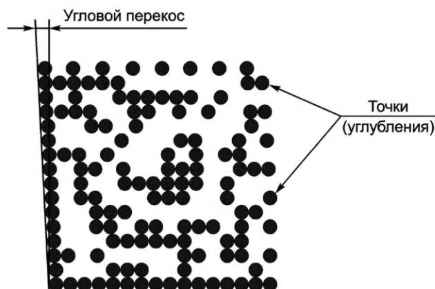
Рисунок 6 — Угловой перекося символа
