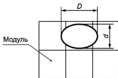
Рисунок 4 — Определение овальности точки
