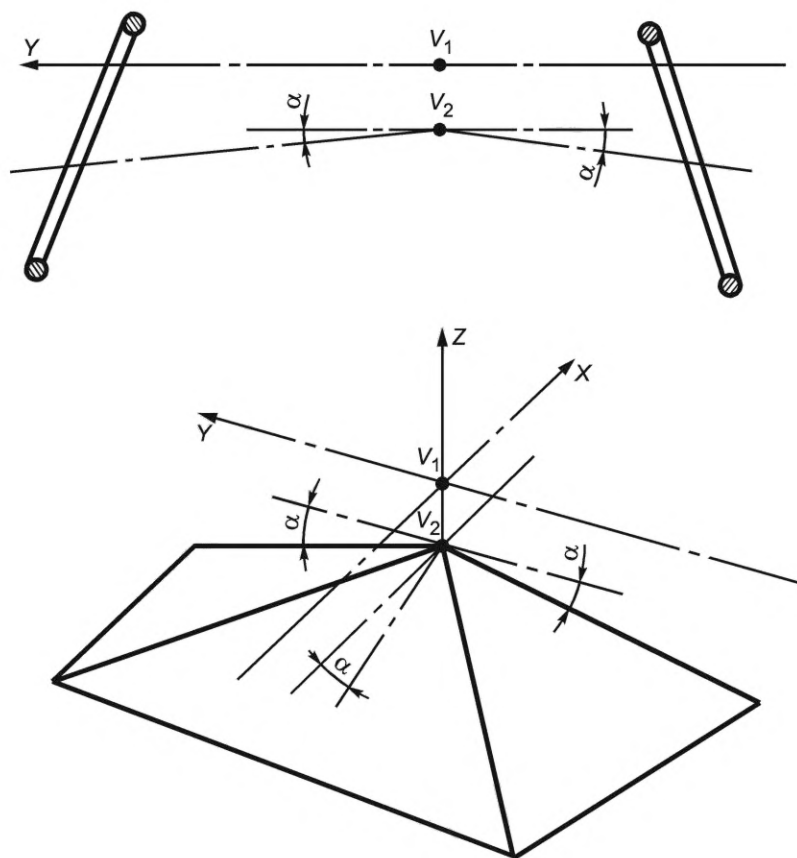
Рисунок Б.7 — Расположение плоскостей, являющихся границами нормативного поля обзора \Pi
