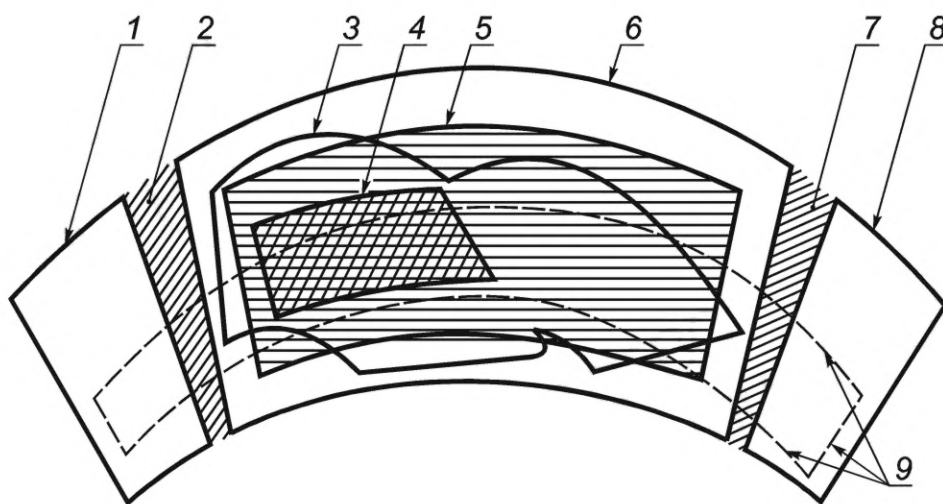
1 — граница прозрачной части левого бокового окна; 2 — левая боковая стойка переднего окна; 3 — контур очистки ветрового стекла; 4 — граница нормативной зоны А; 5 — граница нормативной зоны Б; 6 — граница прозрачной части ветрового стекла; 7 — правая боковая стойка переднего окна; 8 — граница прозрачной части правого бокового окна; 9 — следы от плоскостей, являющихся границами нормативного поля обзора П
