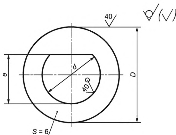
Рисунок И.5 — Шайба для фиксации осей
