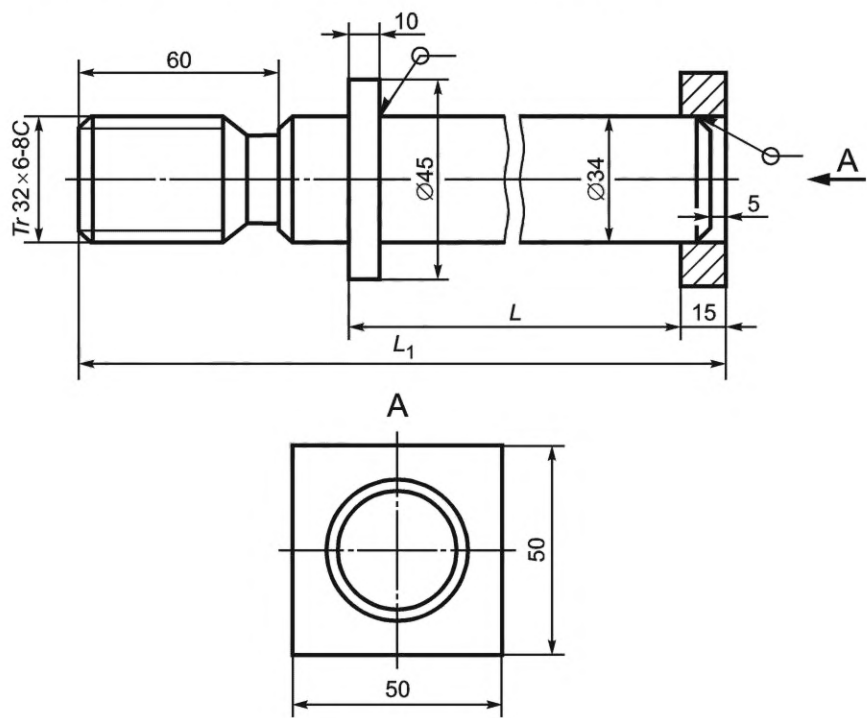
Рисунок И.3 — Болт для стяжек
