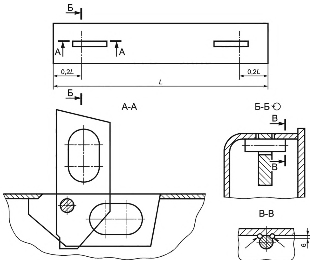
Рисунок Б.2 — Пример установки строповочного устройства в борте
