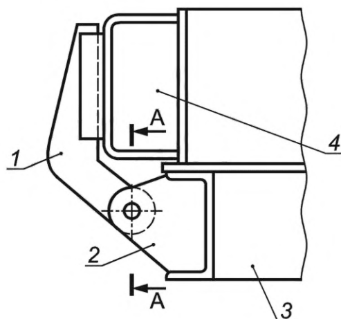
Рисунок К.4 — Шарнирное устройство
