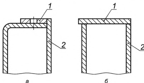
1 — опорная поверхность; 2 — формообразующая поверхность
