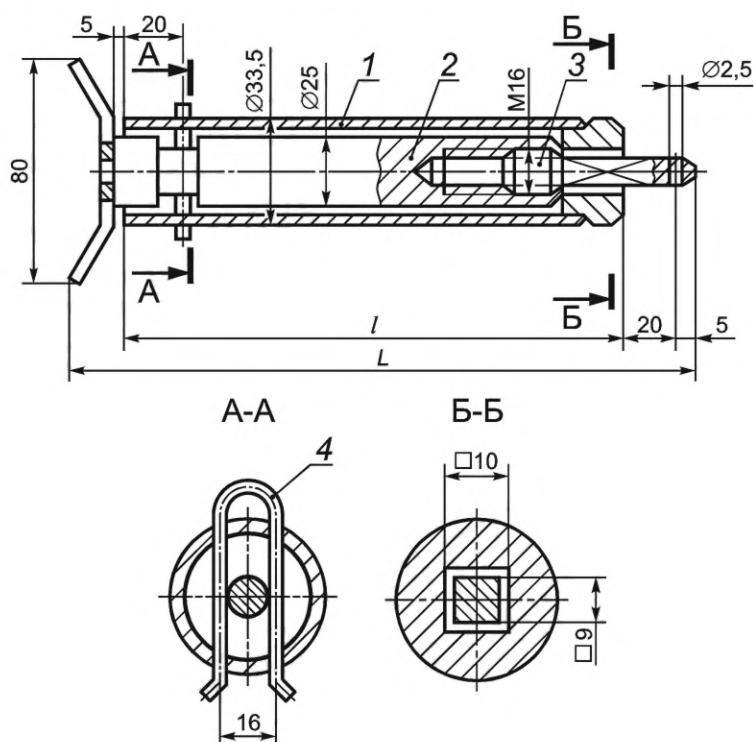
1 — цилиндр; 2 — фиксатор; 3 — винт; 4 — скоба Рисунок Ж.1 — Фиксатор для закладных деталей с квадратным отверстием
