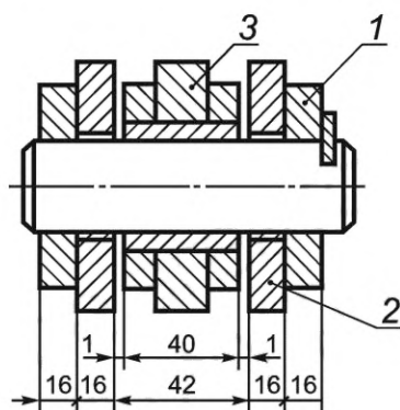
1 — компенсатор; 2 — проушина; 3 — кронштейн
