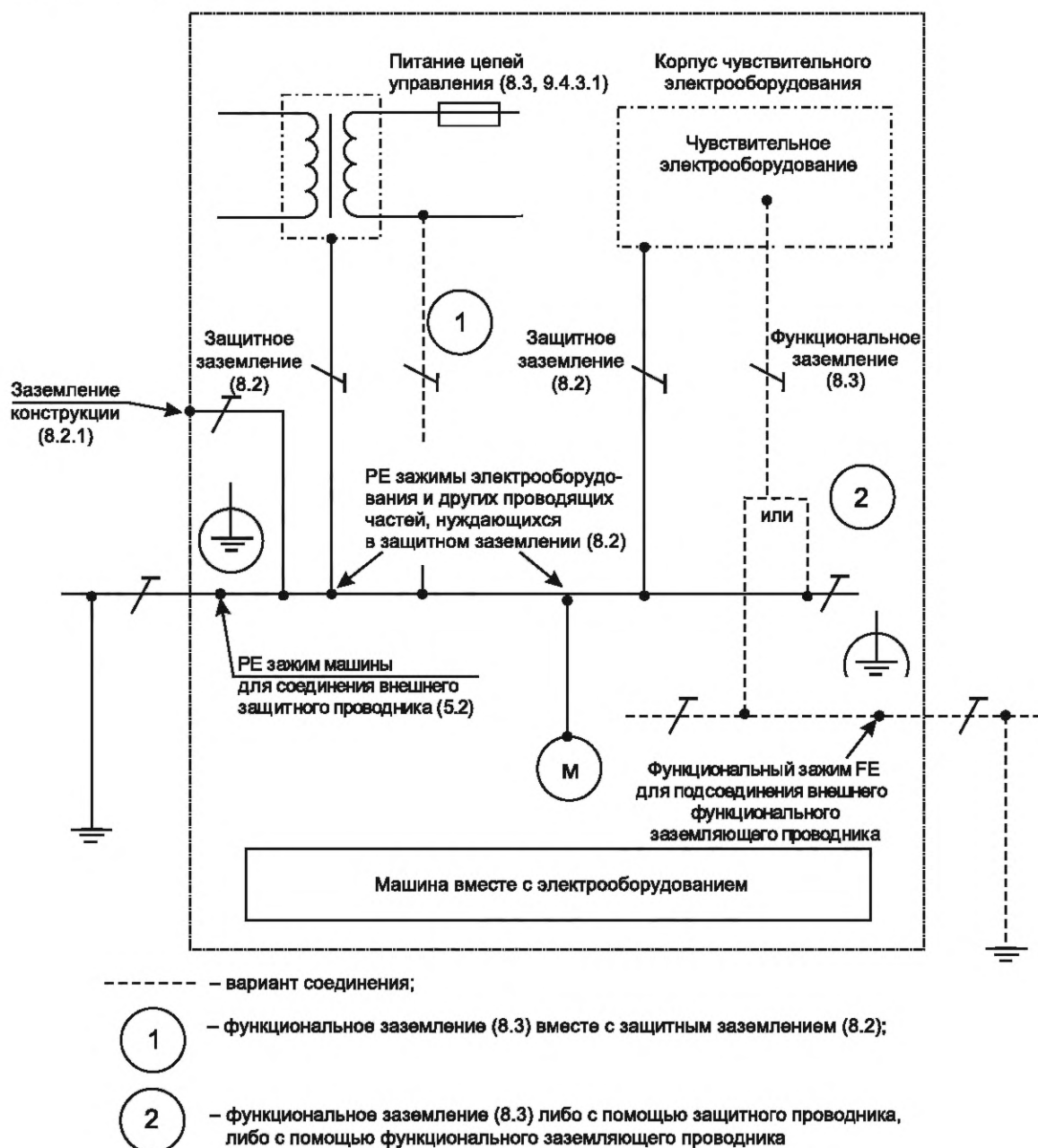
Рисунок 2 — Пример эквипотенциального контура заземления для электрооборудования крана
