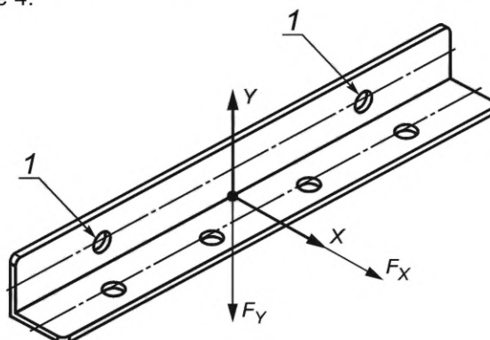
Рисунок 4 — Пример точки опоры и направления сил для проверки прочности
