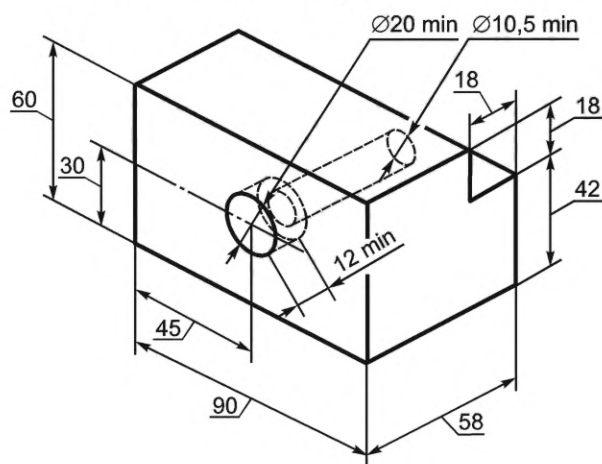
Рисунок 5 — Зацеп типа 1
