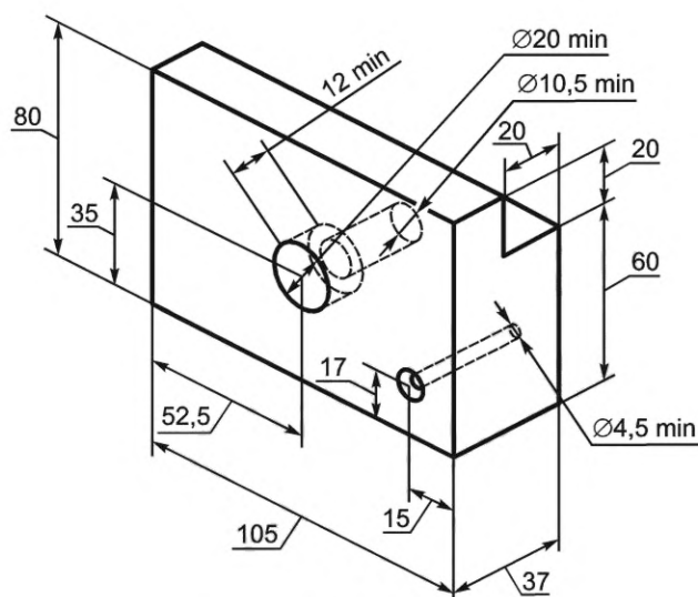
Рисунок 7 — Зацеп типа 3
