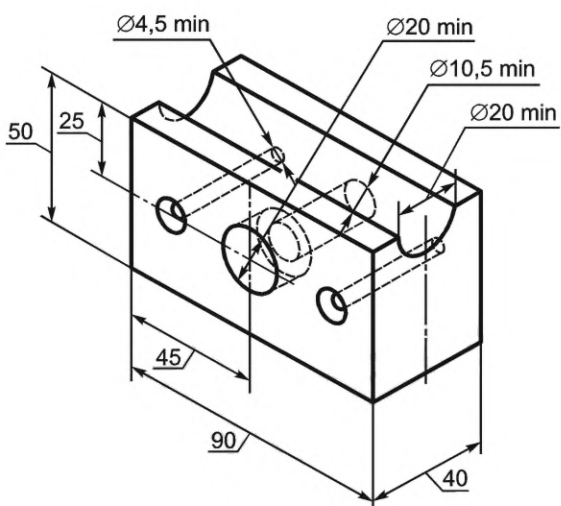
Рисунок 6 — Зацеп типа 2
