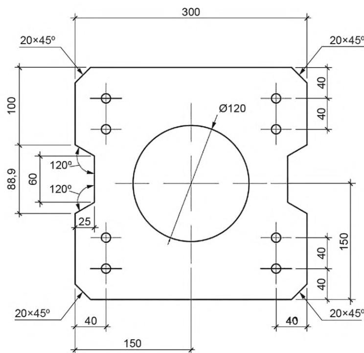
Рисунок 1 — Сечение сваи 30 × 30 см стандартного типа
