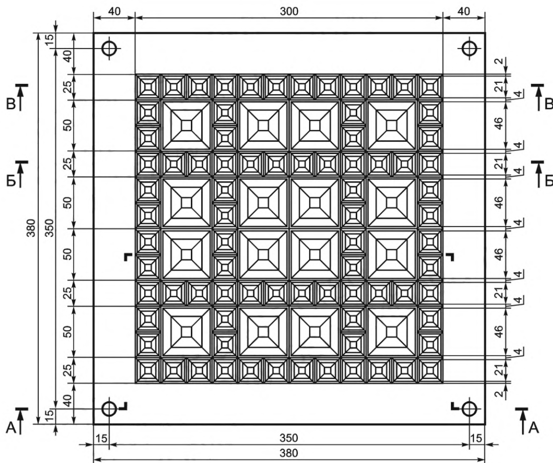
Рисунок А.1 — Щебеночная плита
