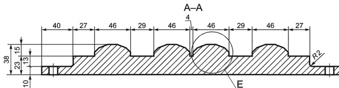
Рисунок А.2 — Сечение А—А
