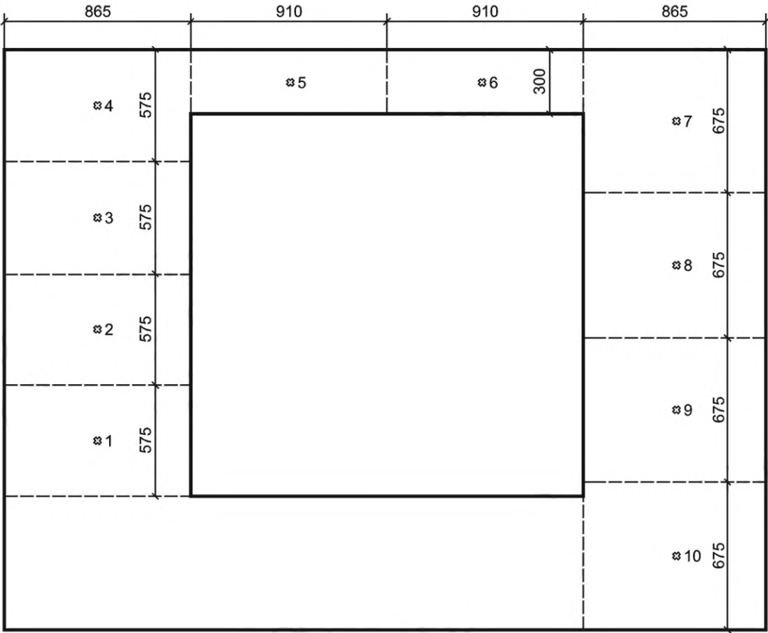
Рисунок А.2 — Схема выбора фрагментов наружных ограждающих конструкций и рекомендуемой расстановки датчиков температуры и тепловых потоков для проведения натурных испытаний
