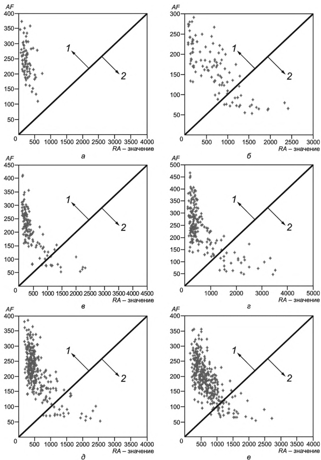
Рисунок Б.1 — Пример классификации активных трещин при нагрузках 15 кН (а), 30 кН (б), 45 кН (в), 60 кН (г), 75 кН (д), 85 кН (е)
