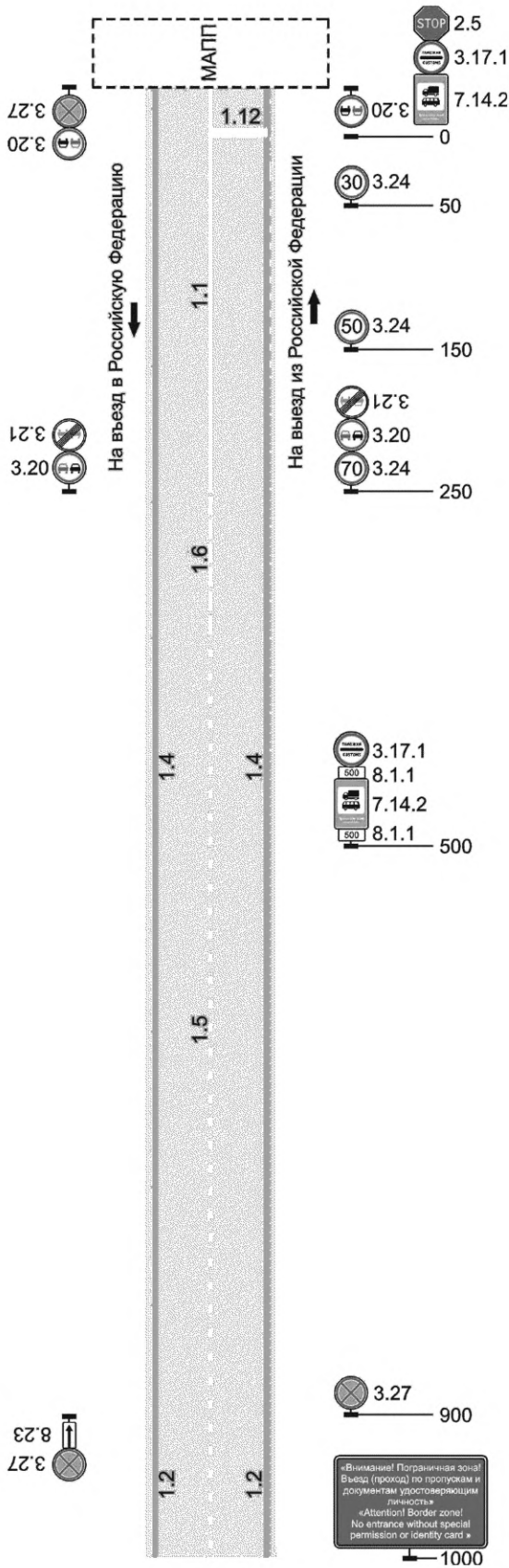
Б.1 Пример схемы примыкания к пункту пропуска со стороны Российской Федерации без полосы ожидания и без распределения транспортного потока приведен на рисунке Б.1.
