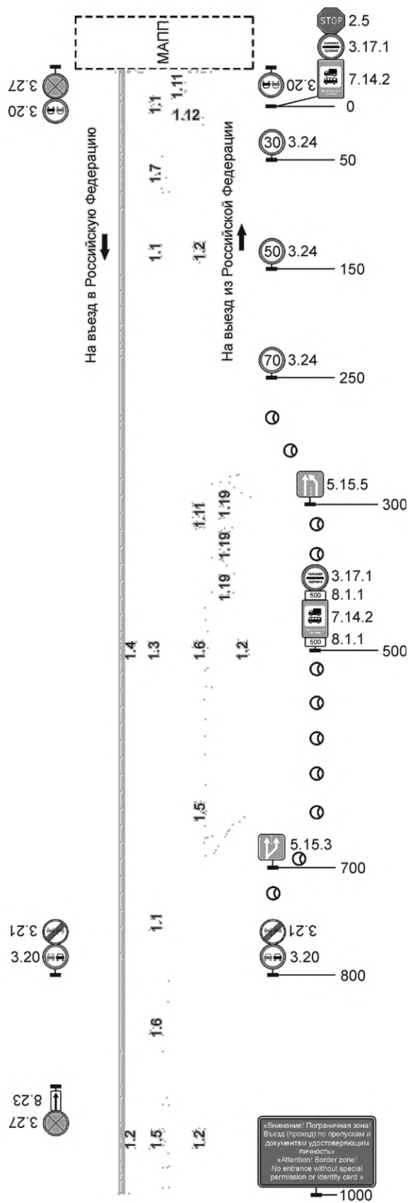
Б.4 Пример схемы примыкания к пункту пропуска со стороны Российской Федерации с полосой ожидания и без распределения транспортного потока приведен на рисунке Б.4.
