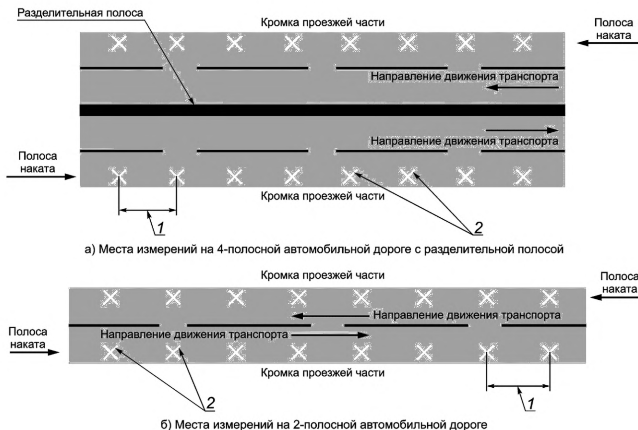
Рисунок Б.1 — Примеры выбора мест измерений в зависимости от количества полос
