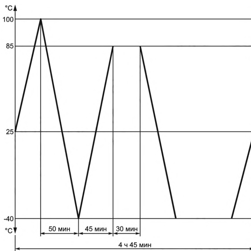
Рисунок 1 — Испытания колесного компонента температурным циклом
