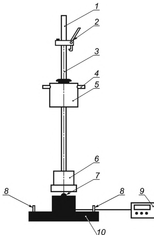
1 — рукоятка; 2 — механизм фиксации и освобождения груза; 3 — направляющая штанга; 4 — ручка падающего груза; 5 — падающий груз; 6 — упругий элемент; 7 — шаровая опора, 8 — ручки для переноски; 9 — электронный регистрирующий блок; 10 — грузочная плита
