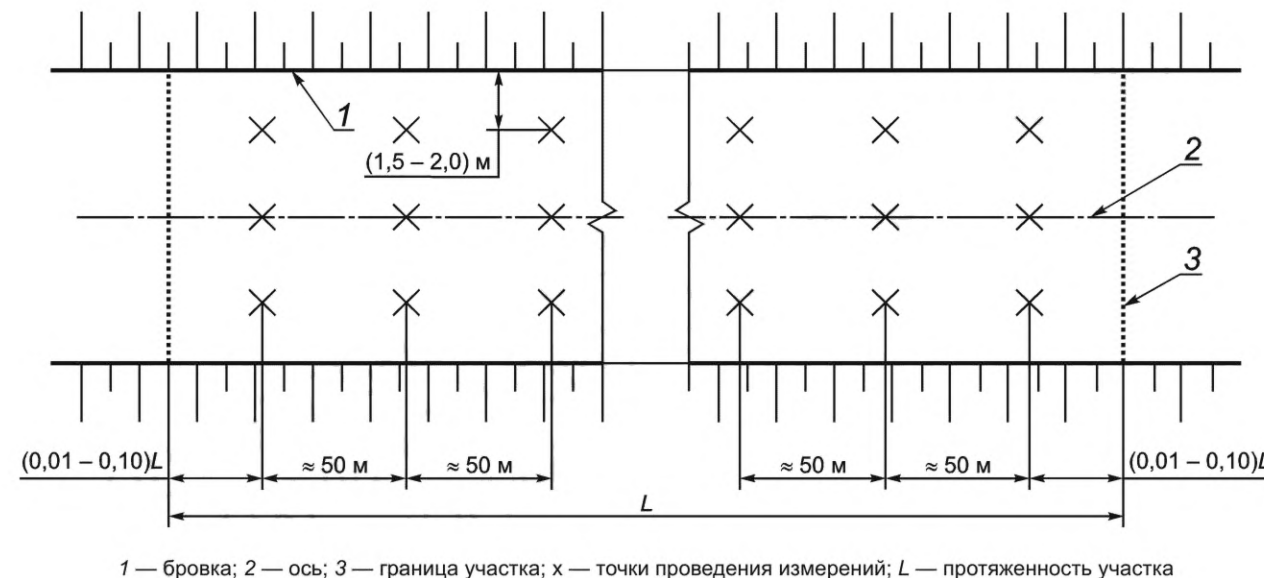
Рисунок 8 — Рекомендуемая схема расположения точек измерения методом динамического нагружения
