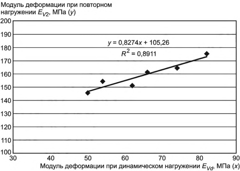
Рисунок Б.1 — График зависимости E_{V2} и E_{Vd}
