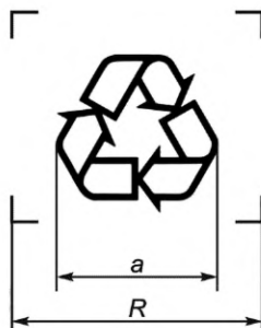
Рисунок Г.2 — Размеры символа переработки
