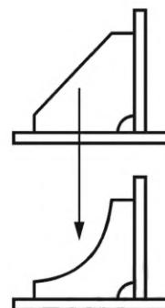
Рисунок 9 — Форма косынок
