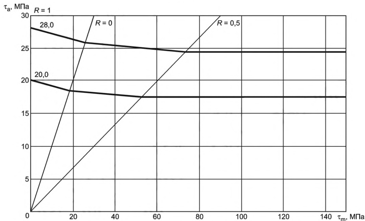
Рисунок 2 — Диаграммы предельных амплитуд цикла для алюминиевых сварных соединений при коэффициенте чувствительности к концентрации напряжений q_\tau = 0,09 материала под воздействием номинальных касательных напряжений
