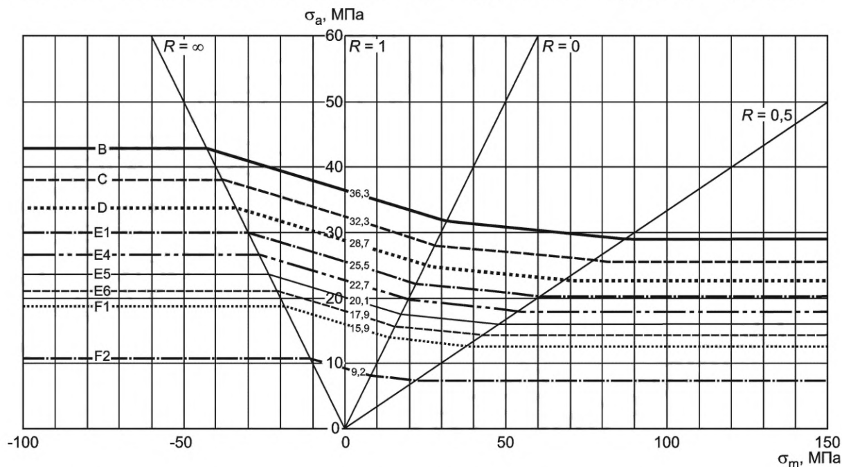
Рисунок 1 — Диаграммы предельных амплитуд цикла для алюминиевых сварных соединений при коэффициенте чувствительности к концентрации напряжений q_\sigma = 0,15 материала под воздействием номинальных нормальных напряжений
