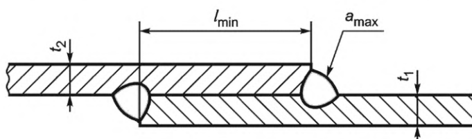
Рисунок 12 — Минимальное расстояние между угловыми швами нахлесточного соединения
