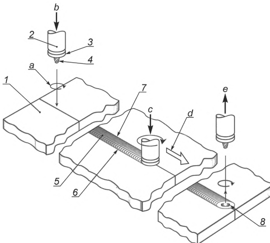
1 — свариваемые детали; 2 — инструмент; 3 — заплечик инструмента; 4 — наконечник инструмента; 5 — лицевая сторона шва; 6 — сторона отставания шва; 7 — сторона набегания шва; 8 — выходное отверстие; a — направление вращения инструмента; b — движение инструмента к детали; c — осевое усилие; d — направление сварки; e — движение инструмента от детали
