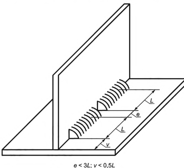
Рисунок 15 — Прерывистые сварные швы
