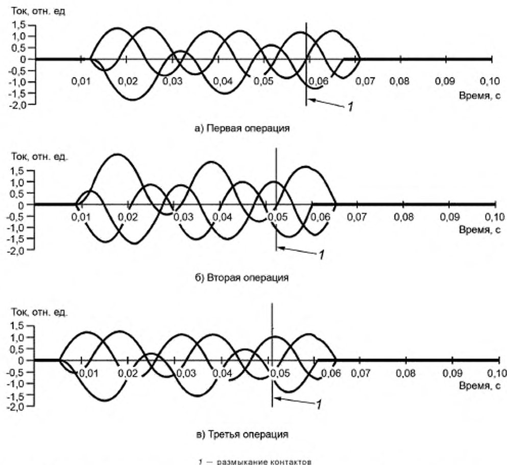
Рисунок 8 — Регулирование моментов инициирования тока и размыкания контактов относительно фазы тока при трехполюсном отключении тока в режиме Т100а
