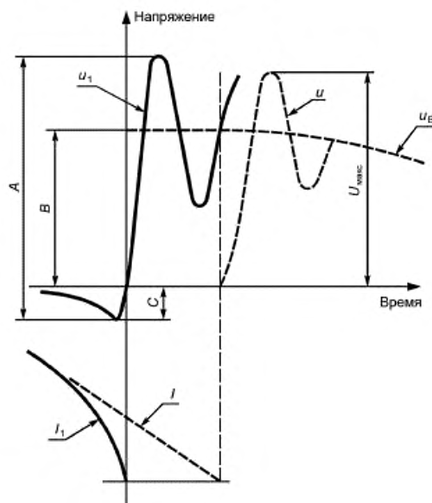
u_1, i_1 — напряжение и ток в опыте; u, i — собственное ПВН и ожидаемый ток, u_B — возвращающееся напряжение
