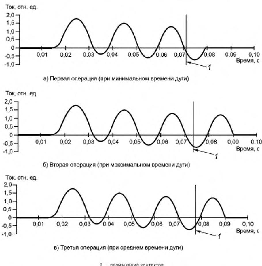
Рисунок 10 — Регулирование моментов инициирования тока и размыкания контактов при однополюсном отключении тока в режиме T100a
