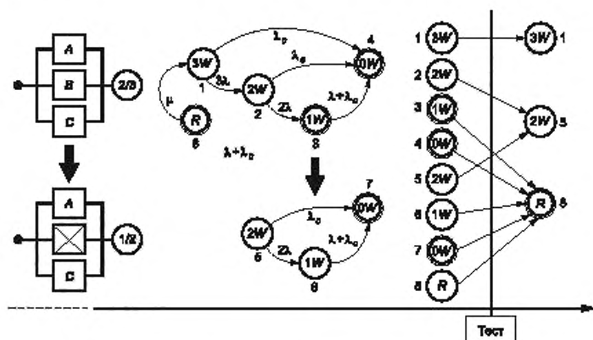
Рисунок Б.30 — Изменение логики (с 2003 на 1002) вместо ремонта первого отказа
