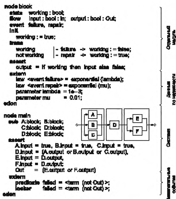
Рисунок Б.37 — Пример моделирования свойств корректно и некорректно функционирующих систем с использованием формального языка
