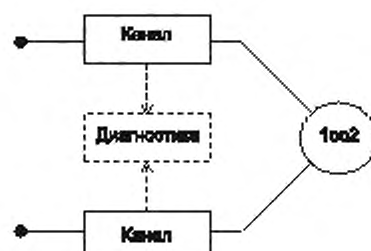
Рисунок Б.8 — Структурная схема архитектуры 2oo2
