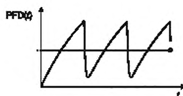
Рисунок Б.25 — Зубчатая кривая, полученная с помощью многофазного марковского подхода
