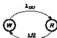
Рисунок Б.26 — Приближенная модель Маркова
