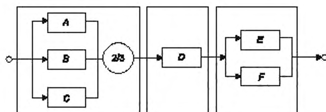
Рисунок Б.16 — Блок-схема надежности простой полной СБЗС системы с датчиками, организованной по схеме 2003
