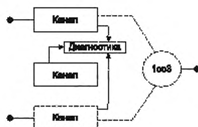
Рисунок Б.12 — Структурная схема архитектуры 2oo3
