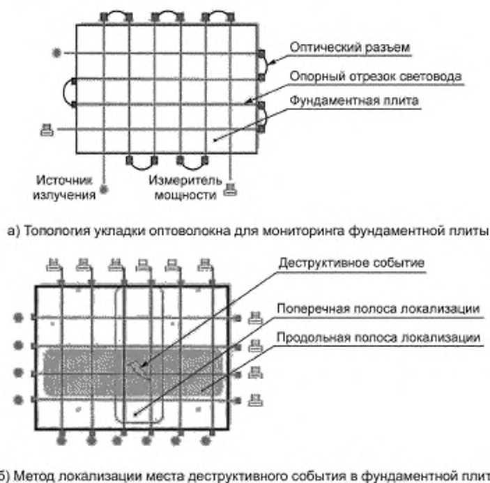
Рисунок 14 — Пример мониторинга деформаций в фундаментной плите с использованием оптоволокон
