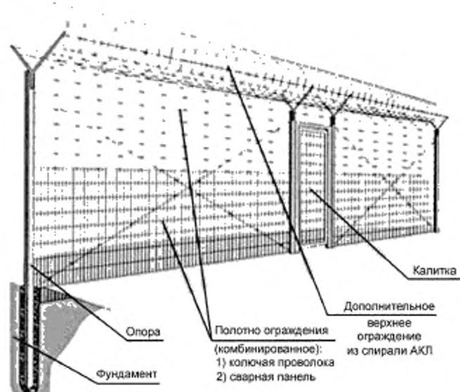
Рисунок 3 — Типовая конструкция и элементы защитного ограждения
