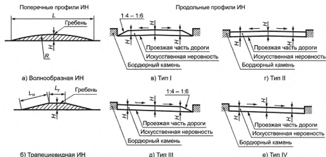
Рисунок 10 — Примеры искусственных неровностей (ИН)
