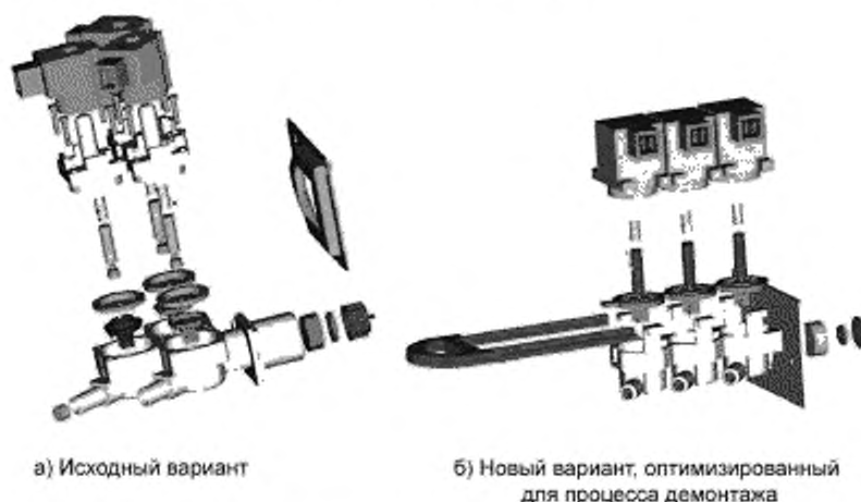
Рисунок А.5 — Иллюстрации конструкции блока клапанов
