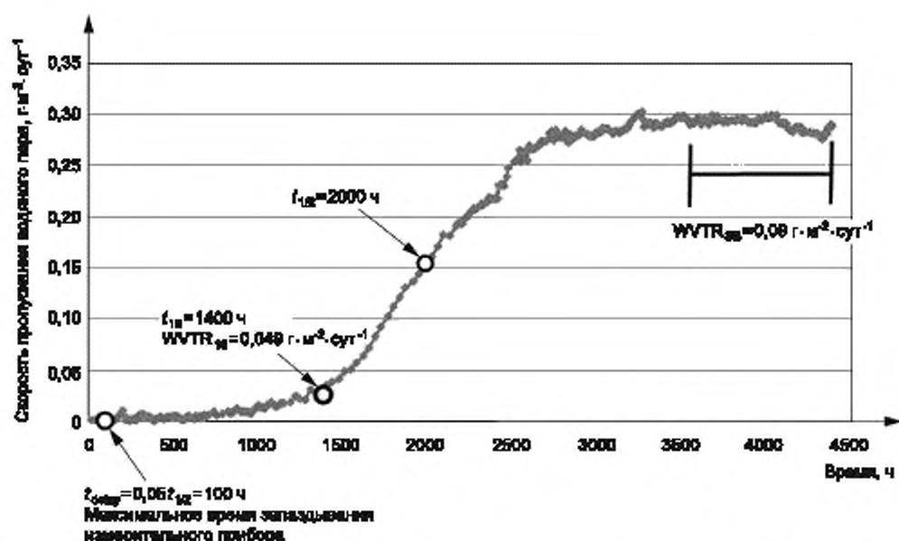
Рисунок А.3 — Пример нефиковской диффузии в полиизобутилене с осушителем, применяемом в качестве материала торцевого уплотнения при температуре внутри испытательной ячейки 38^\circ\text{C} , относительной влажности в камере источника влаги 100 % и толщине образца 1 мм
