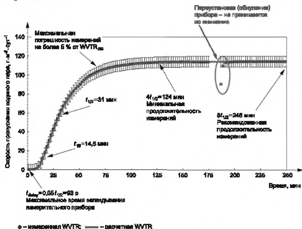
Рисунок А.1 — Пример фиковской диффузии в пленке ЭВА при температуре внутри испытательной ячейки 85 °С, относительной влажности в камере источника влаги 100 % и толщине образца 2,84 мм
