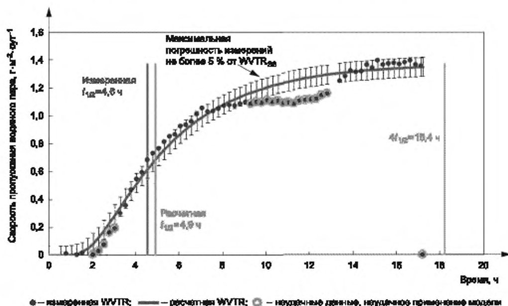
Рисунок А.2 — Пример неудачных измерений пленки ПЭТФ при температуре внутри испытательной ячейки 22 °С, относительной влажности в камере источника влаги 100 % и толщине образца 0,018 мм
