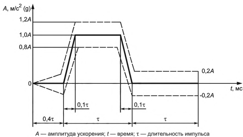
Рисунок А.3 — Трапецеидальный импульс ударного воздействия
