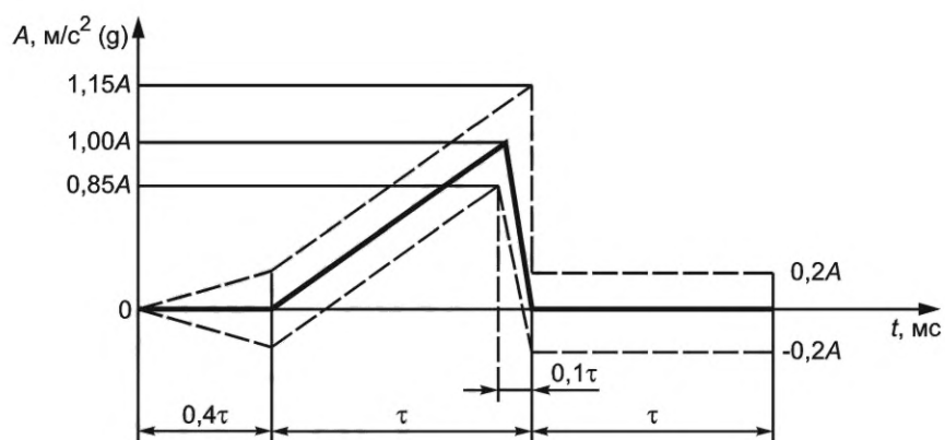
Рисунок А.2 — Треугольный (пилообразный) импульс ударного воздействия
