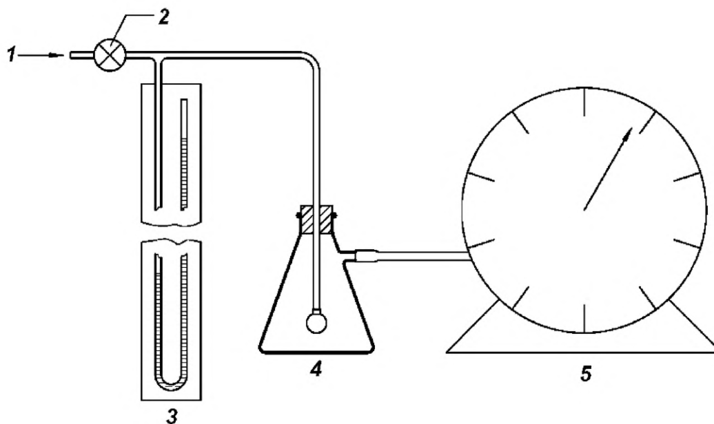
1 — чистый сухой воздух; 2 — регулятор; 3 — водяной манометр; 4 — фильтровальная колба; 5 — счетчик газа
