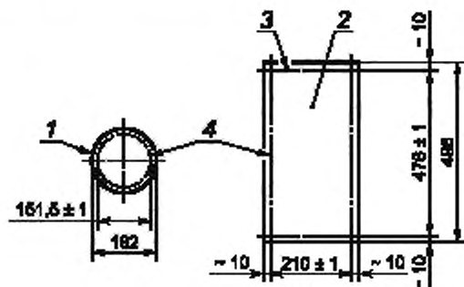
1 — две круглые части; 2 — боковая поверхность; 3 — продольный шов; 4 — торцевой шов
