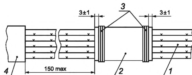
Рисунок 6.2 — Установка поливинилхлоридной или резиновой бирки на жгут
