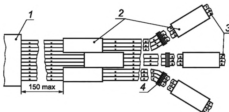
Рисунок 6.4 — Установка поливинилхлоридных или резиновых бирок при заделке нескольких жгутов в электрический соединитель
