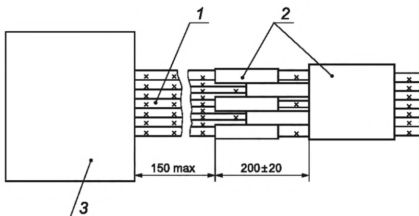
1 — жгут; 2 — термоусаживаемая бирка; 3 — электрический соединитель
