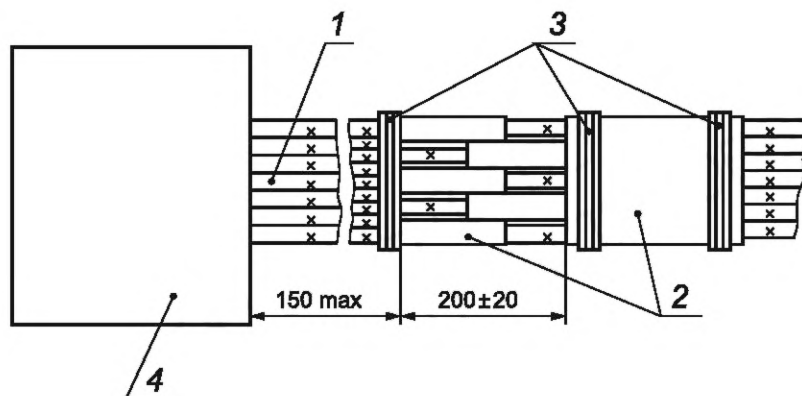
1 — жгут; 2 — поливинилхлоридная или резиновая бирка; 3 — бандаж; 4 — соединитель электрический
