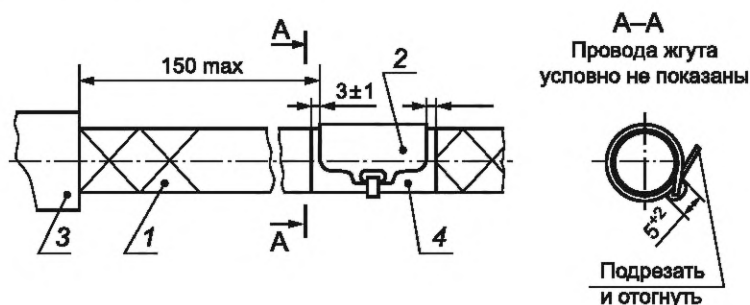
Рисунок 6.6 — Установка металлических бирок на экранированные жгуты
