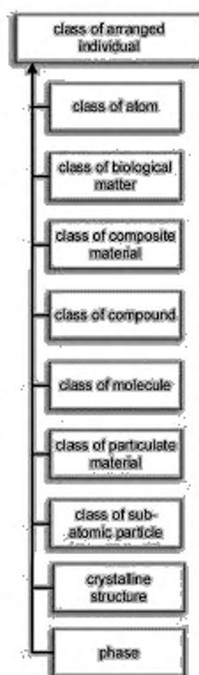
Рисунок Е.6 — Подклассы представляющего классы упорядоченных индивидов класса class of arranged individual
