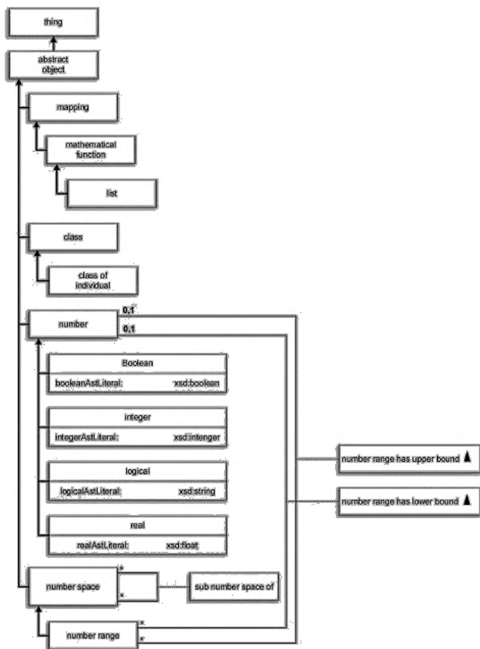
Рисунок Е.8 — Основные подклассы представляющего абстрактные объекты класса abstract object
