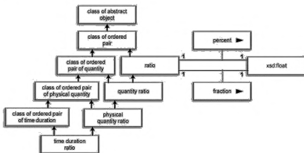
Рисунок Е.13 — Классы, связанные с представляющим класс упорядоченных пар классом class of ordered pair и представляющим соотношение классом ratio
