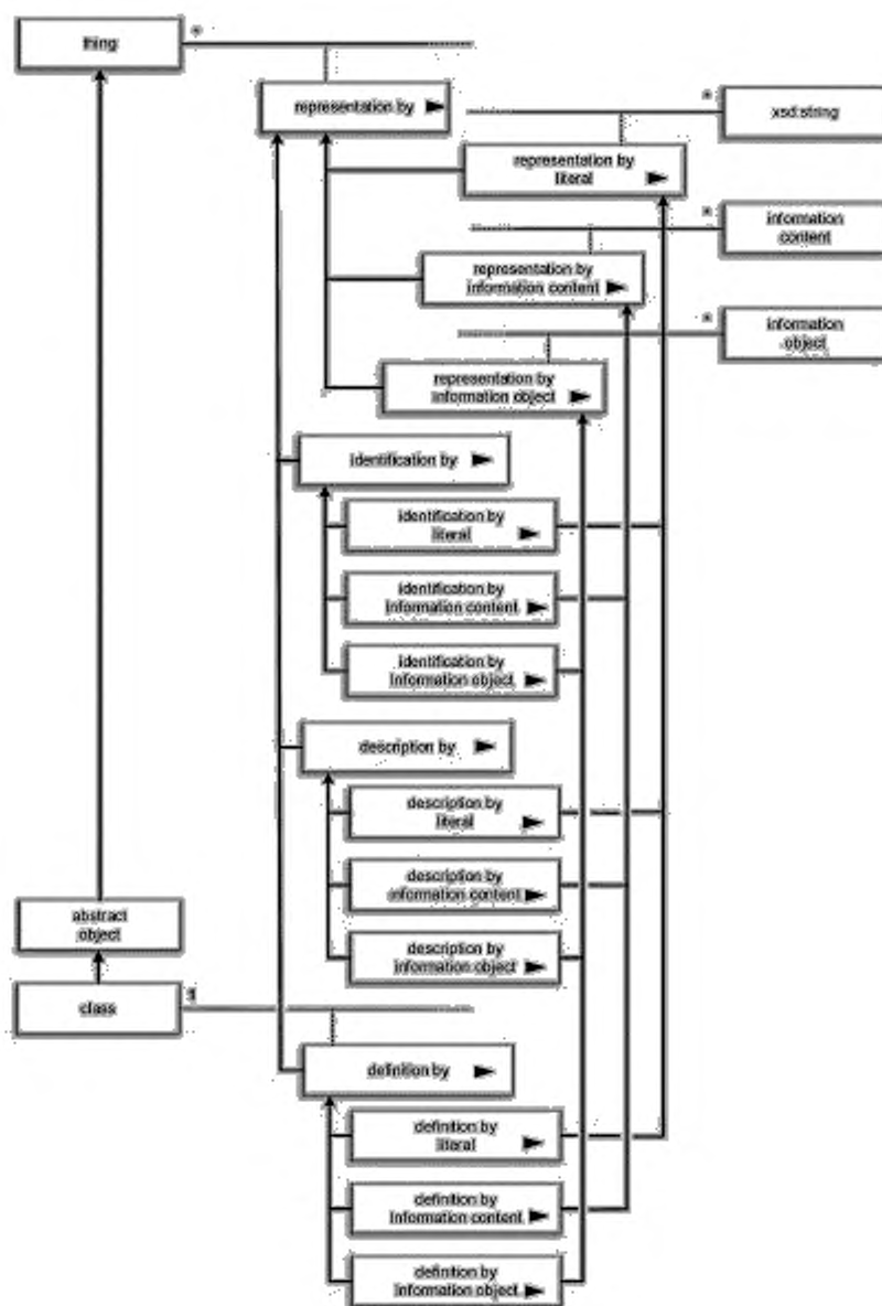
Рисунок Е.17 — Используемые для обозначения, описания и определения подтипы представляющего ссылку на представление свойства representation by
