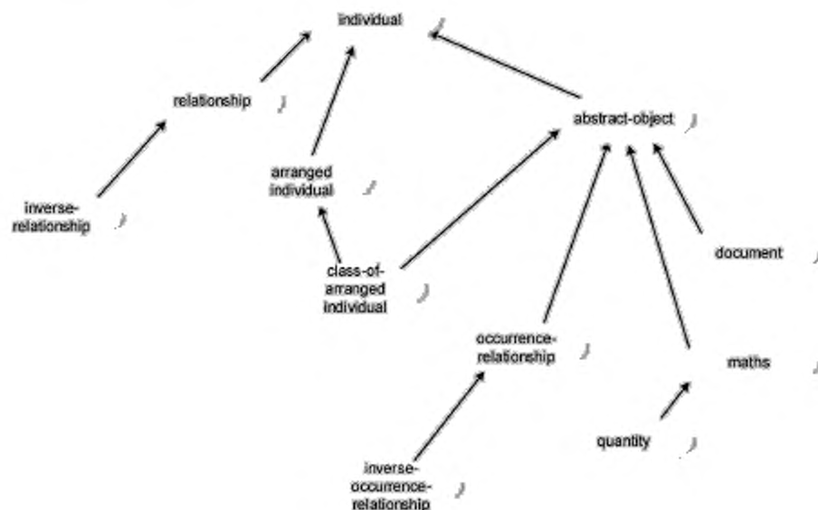
Рисунок А.1 — Иерархия импорта
