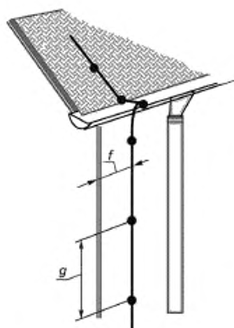
в) Установка токоотвода с присоединением к водосточному желобу
