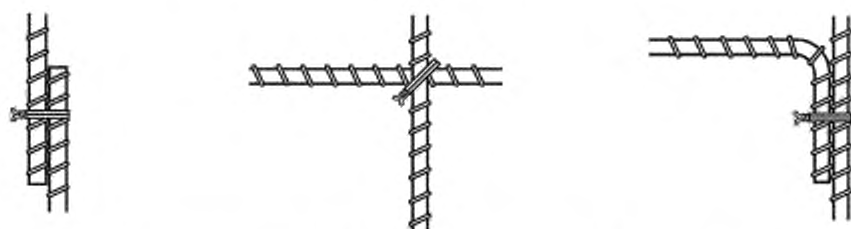
г) Соединения с помощью вязки, пригодные только для целей ЭМС
