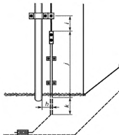
г) Установка испытательного зажима на токоотводе и соединение с водосточной трубой
