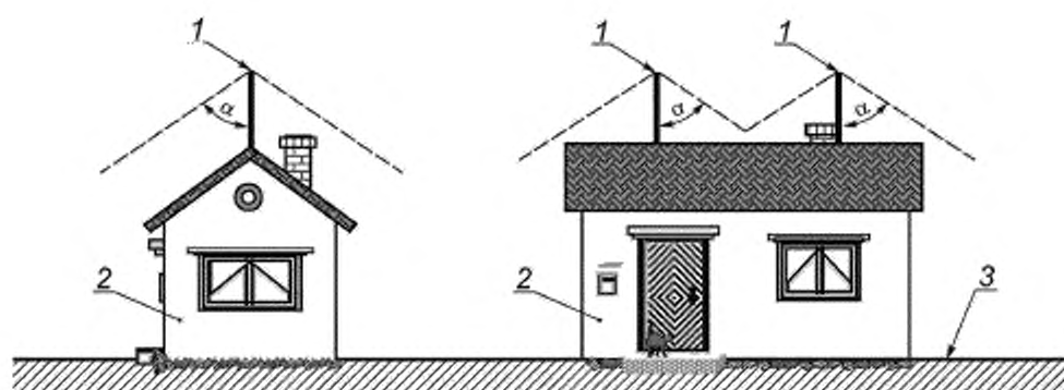
б) Пример использования двух стержневых молниеводводов
