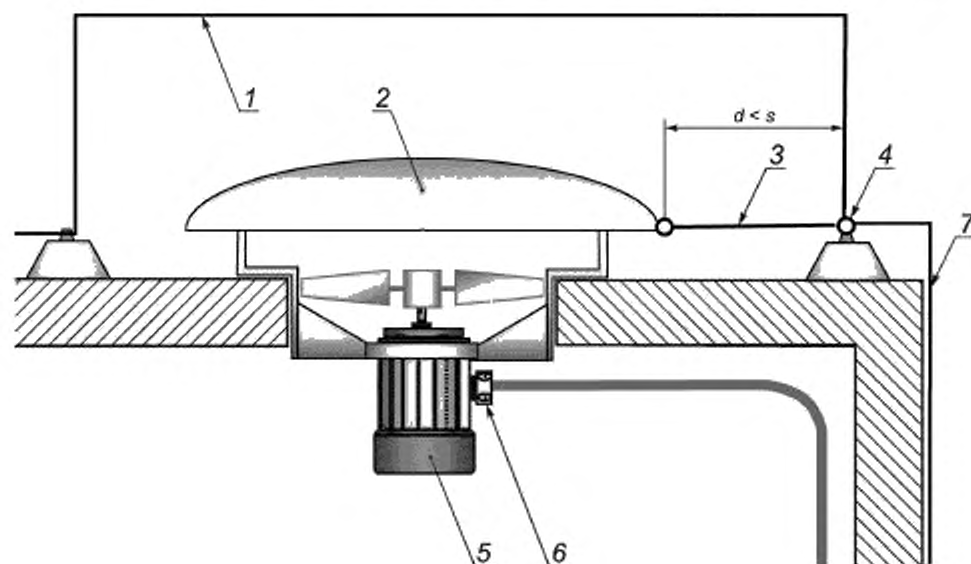
1 — проводник молниеприемника; 2 — металлическая крышка; 3 — проводник уравнивания потенциалов; 4 — горизонтальный проводник молниеприемника; 5 — электрическое оборудование; 6 — электрическая клеммная коробка с устройством защиты от перенапряжения; 7 — токоотвод
