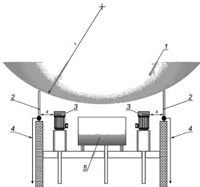
r — катящаяся сфера; 2 — стержневой молниеприемник; 3 — электрическое оборудование; 4 — токоотвод; 5 — металлический резервуар; r — радиус катящейся сферы (см. таблицу 2); s — разделительное расстояние в соответствии с 6.3
