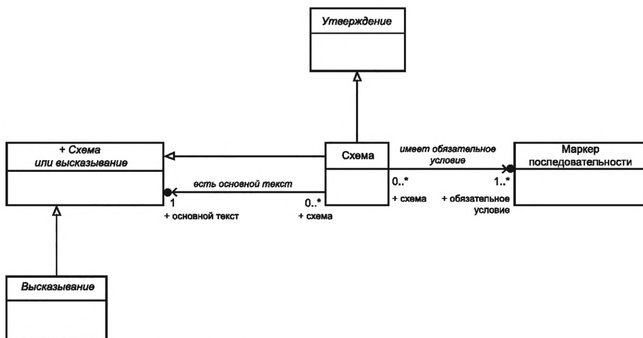
Рисунок 9 — Абстрактный синтаксис текстовых конструкций
