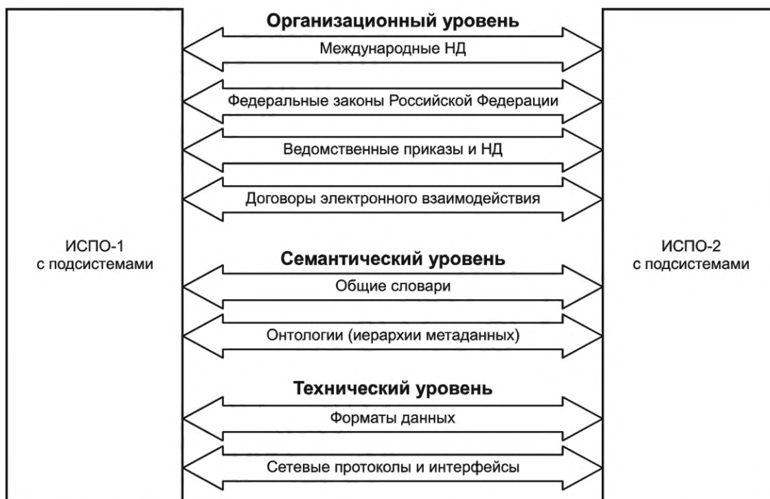
Рисунок 4 — Проблемно-ориентированная модель интероперабельности информационных систем предметных областей
