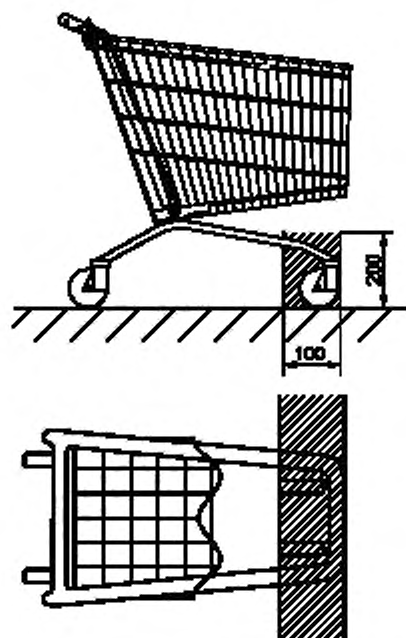
Рисунок В.10 — Пространство для испытания
