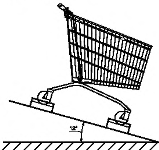
Рисунок Г.2 — Положение тележки на испытательной платформе
