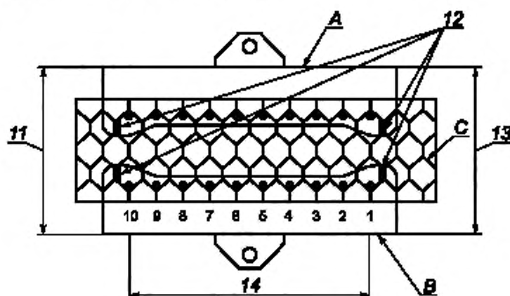
1 — 10 — стальные крючки; 11 — левое измеряемое значение; 12 — боковые крючки; 13 — правое измеряемое значение; 14 — фактическая ширина А — верхняя стальная пластина; В — нижняя стальная пластина; С — образец проволоочной сетки
