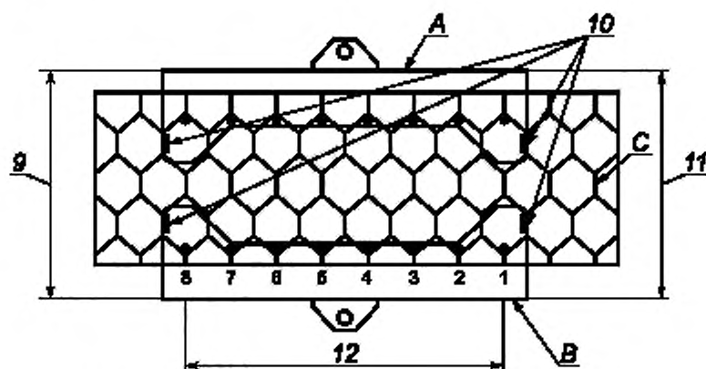
7—8 — стальные крючки; 9 — левое измеряемое значение; 10 — боковые крючки; 11 — правое измеряемое значение; 12 — фактическая ширина A — верхняя стальная пластина; B — нижняя стальная пластина; C — образец проволоочной сетки
