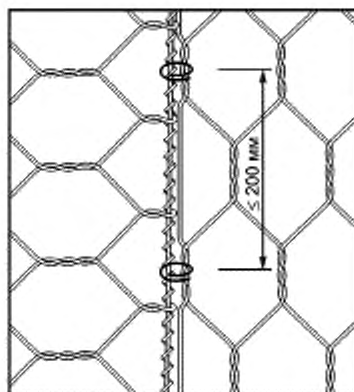
Рисунок 7 — С-образные кольца
