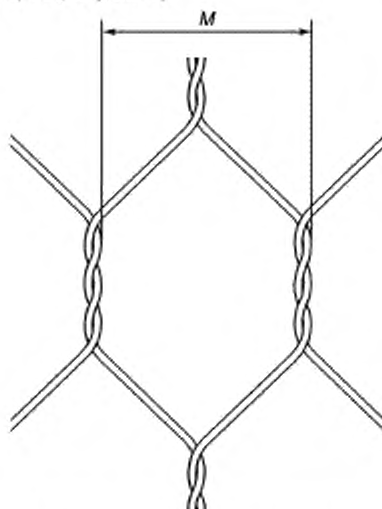
Рисунок 1 — Размер ячеек
