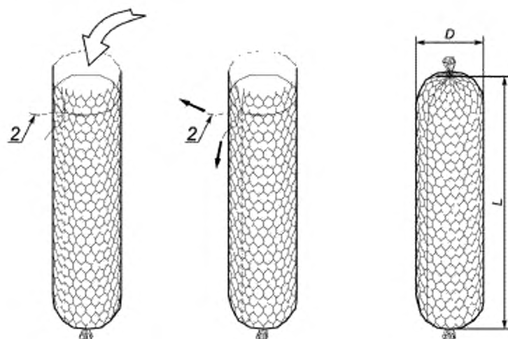
\Gamma — наполнение; 2 — соединяющая проволока; D — диаметр каменного вальца; L — длина каменного вальца
