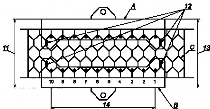
1—10 — стальные крючки; 11 — левое измеряемое значение; 12 — боковые крючки; 13 — правое измеряемое значение; 14 — фактическая ширина А — верхняя стальная пластина; В — нижняя стальная пластина; С — образец проволочной сетки
