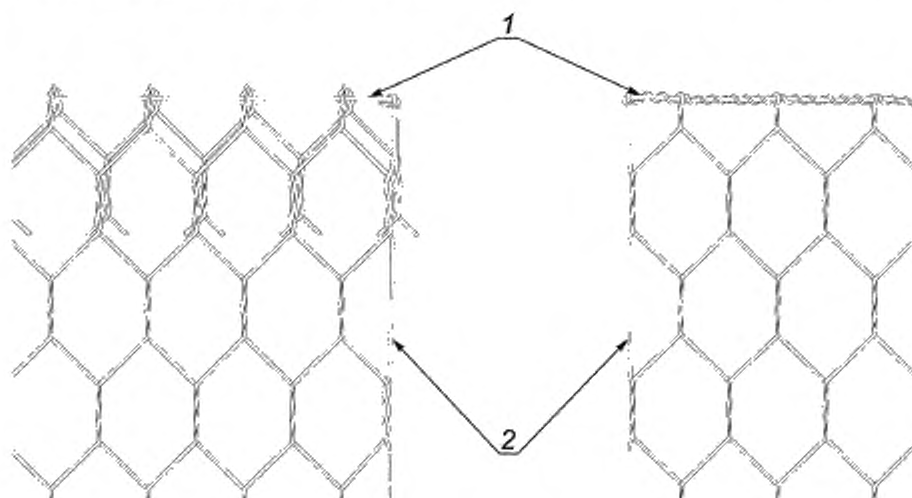
1 — продольная бортовая проволока, 2 — поперечная бортовая проволока
