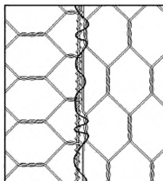
Рисунок 6 — Крепежная проволока
