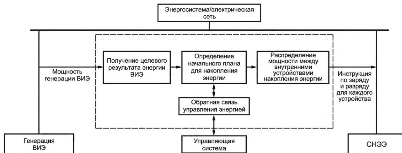
Рисунок 34 — Пример основных процедур сглаживания мощности стохастической генерации ВИЭ
