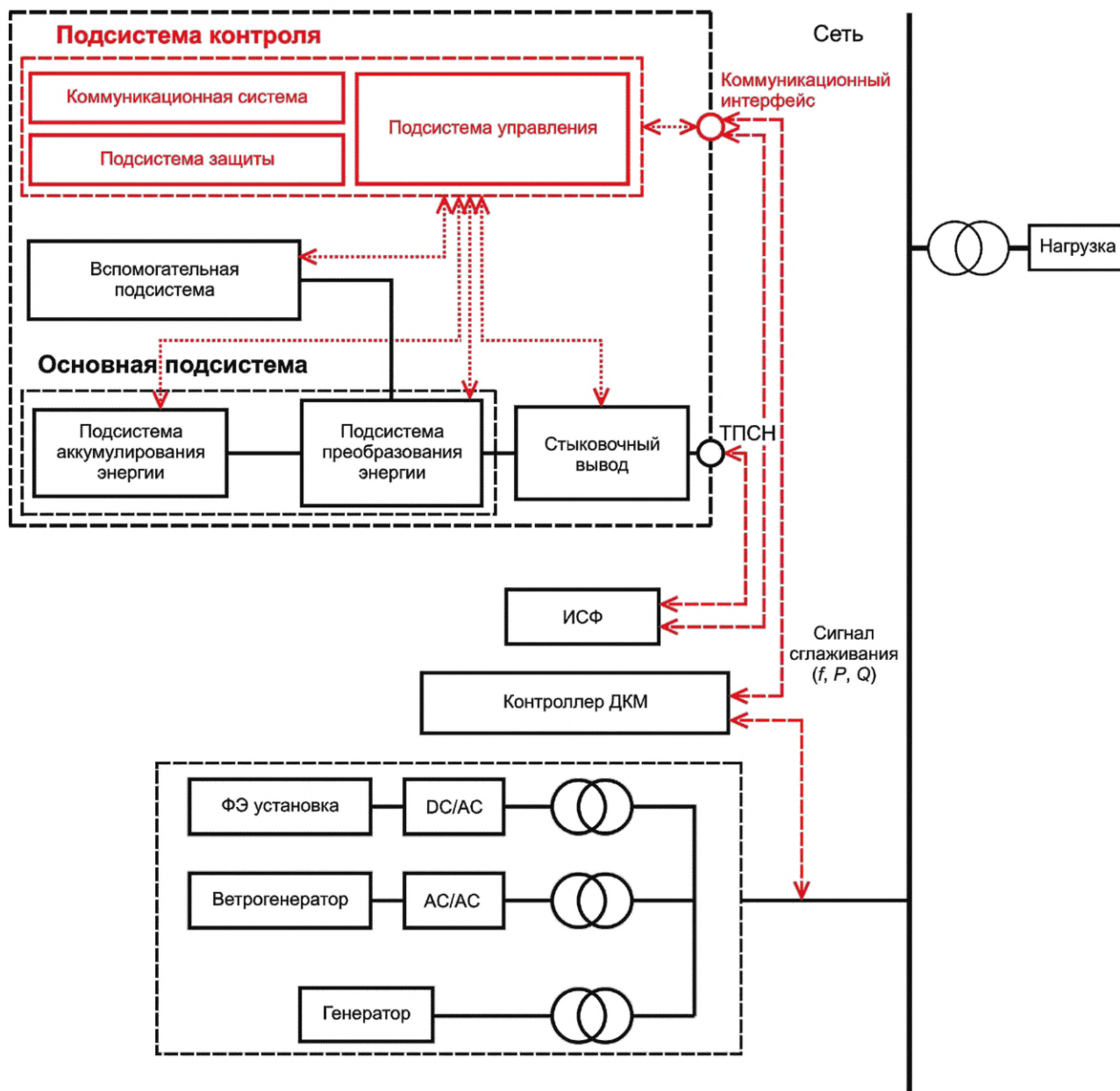
Рисунок 45 — Пример архитектуры СНЭЭ для ДКМ
