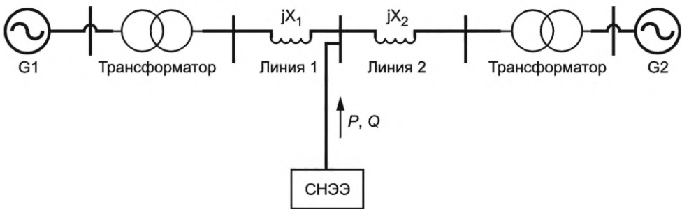
Рисунок 42 — Пример архитектуры одиночной несекционированной системы шин, подключенной к СНЭЭ
