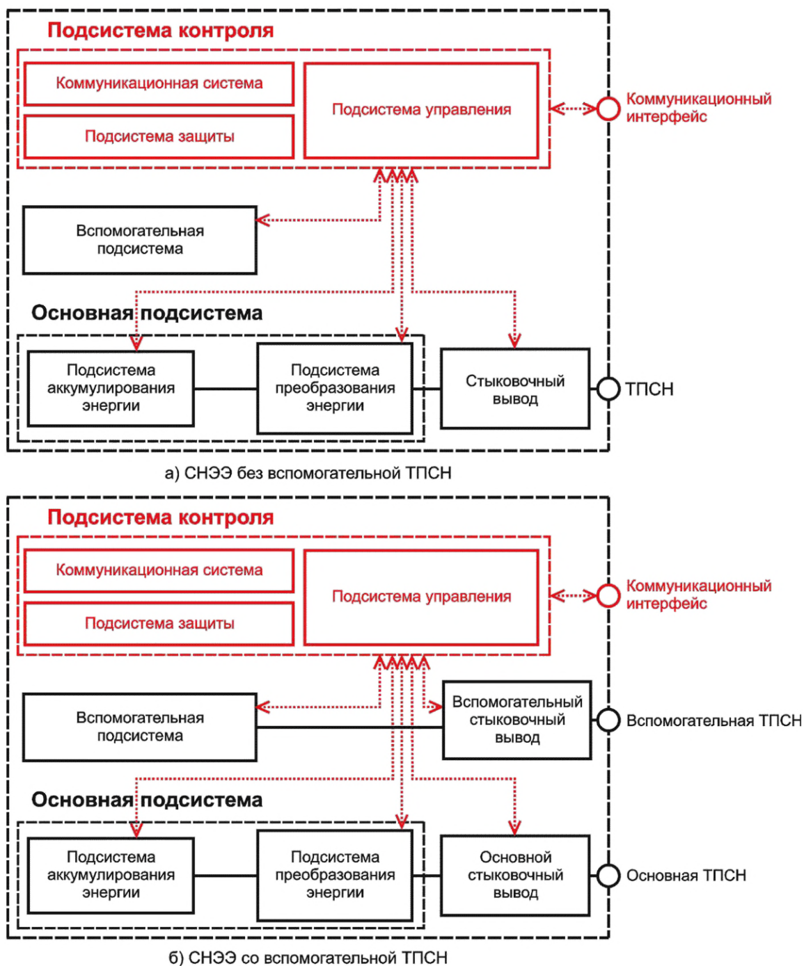
Рисунок 1 — Примеры архитектуры СНЭЭ
