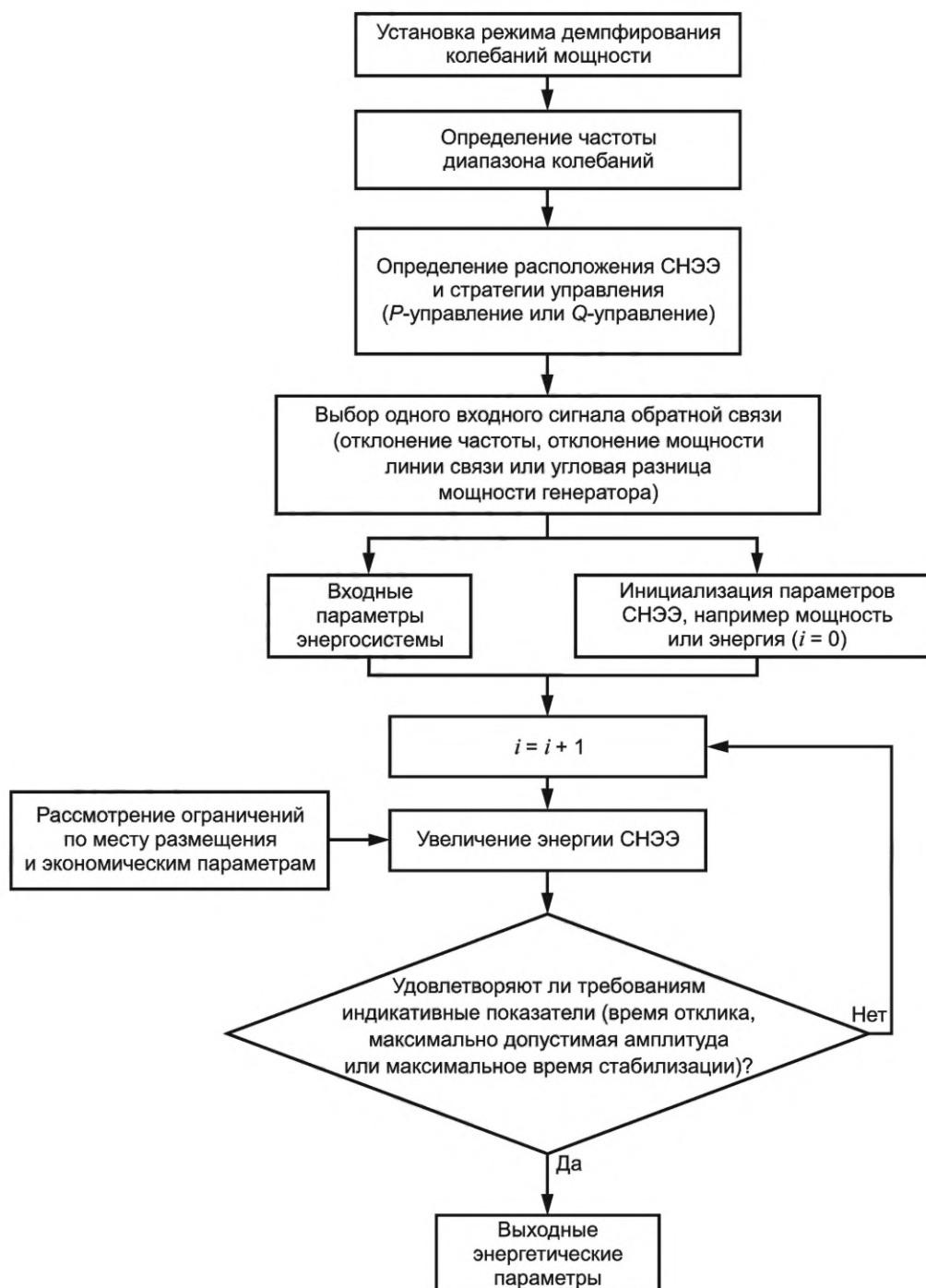
Рисунок 46 — Пример процесса расчета энергетических параметров СНЭЭ для применения ДКМ
