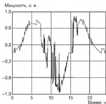
Рисунок А.7 — Пример изменения реактивной мощности СНЭЭ в ТПН [5]
