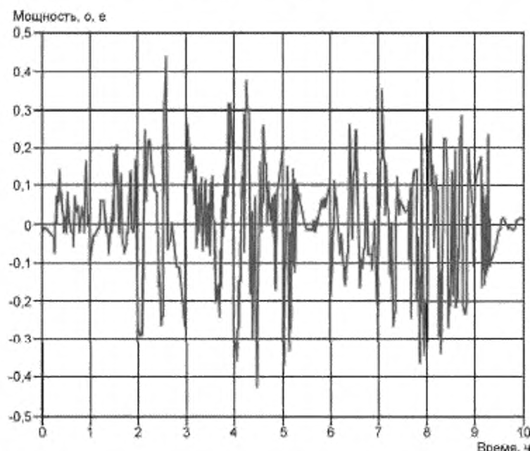
Рисунок А.5 — Пример графика входной и выходной мощности СНЭЭ для приложения сглаживания графика мощности фотоэлектрической панели [5]
