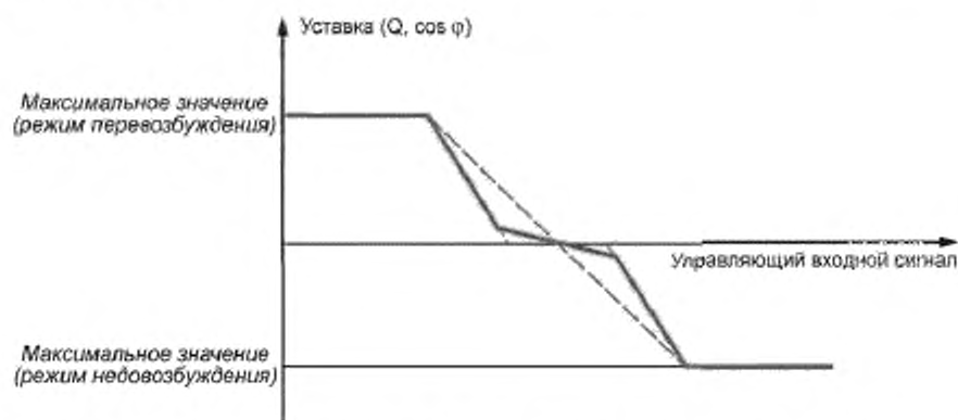
Рисунок 10 — Пример типовой характеристики регулирования [3], [4]
