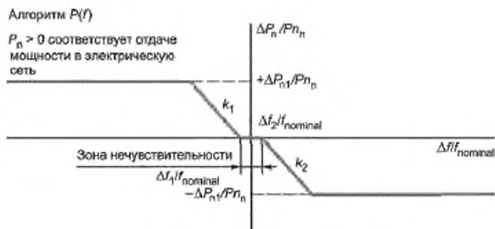
Рисунок 6 — Пример алгоритма P(f)
