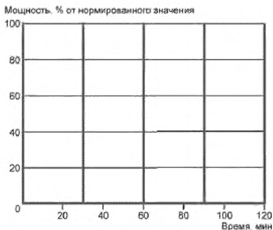
Рисунок А.1 — Пример рабочего цикла приложения резервирования функции первичного регулирования частоты сети [5]
