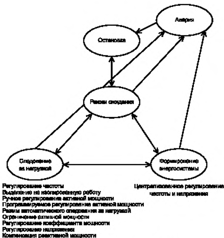
Рисунок 5 — Пример рабочих режимов СНЭЭ
