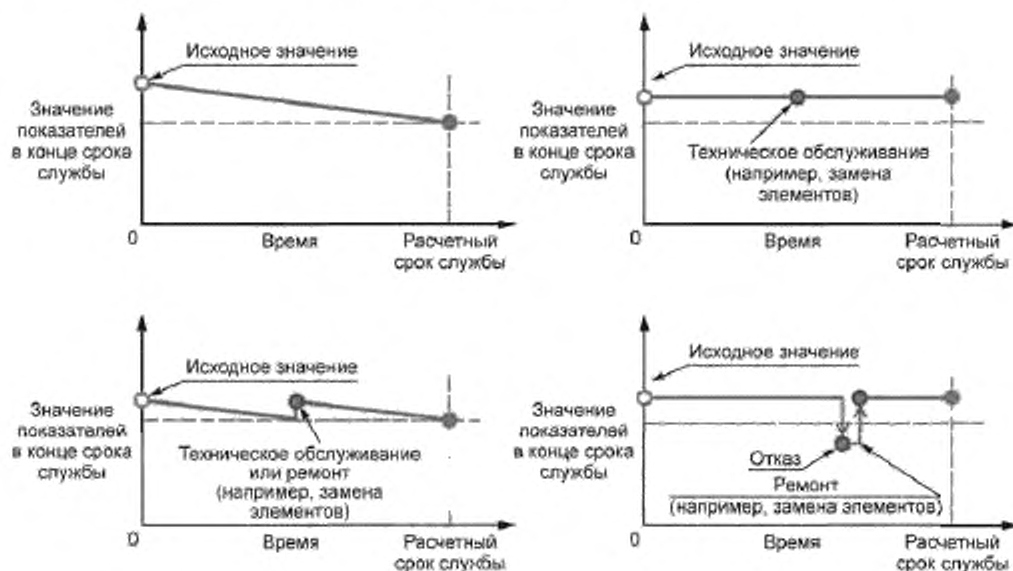
Рисунок 4 — Факторы, учитываемые при определении расчетного срока службы СНЭЭ
