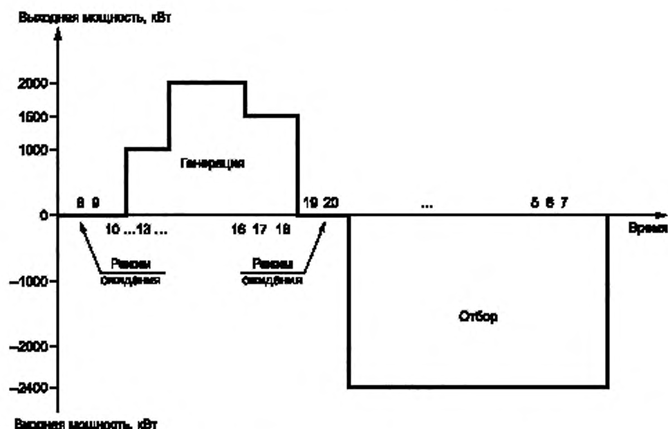
Рисунок 8 — Пример суточного рабочего графика в основной ТПН
