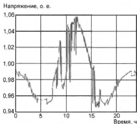
Рисунок А.6 — Пример изменения напряжения в ТПН [5]
