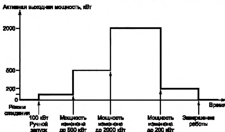
Рисунок 7 — Пример ручного регулирования активной выходной мощности в основной ТПН
