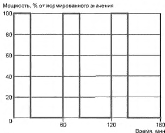
Рисунок А.2 — Пример рабочего цикла приложения резервирования функции вторичного регулирования частоты сети [4]
