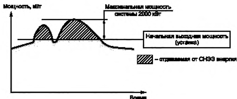
Рисунок 9 — Пример покрытия пиковых нагрузок
