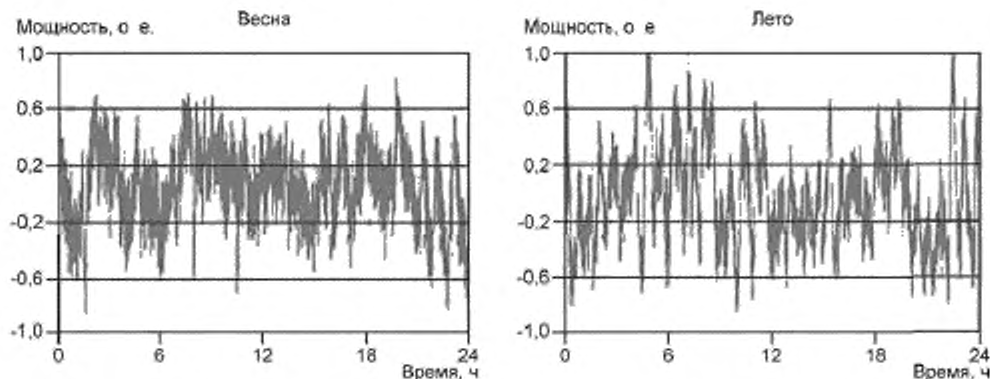
Рисунок А.3, лист 1 — Пример значений входной и выходной мощности СНЭЭ в режиме выполнения приложения непрерывного регулирования частоты сети для четырех сезонов года [5]
