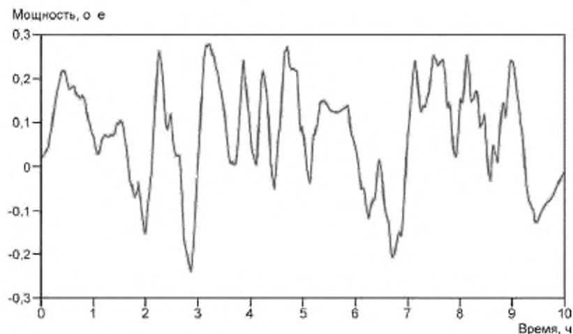
Рисунок А.4 — Пример графика входной и выходной мощности СНЭЭ для приложения обеспечения надежности работы фотоэлектрической генерации [5]
