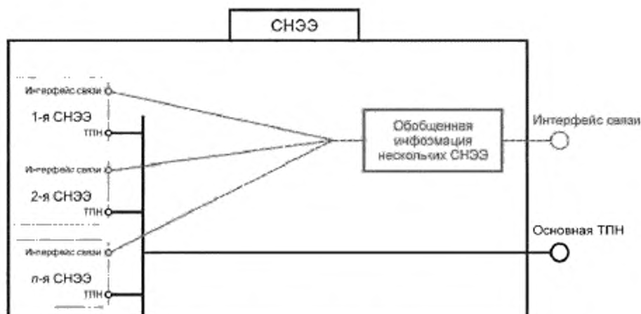
Рисунок 12 — Совокупность нескольких СНЭЭ, подсоединенных к одной ТПН
