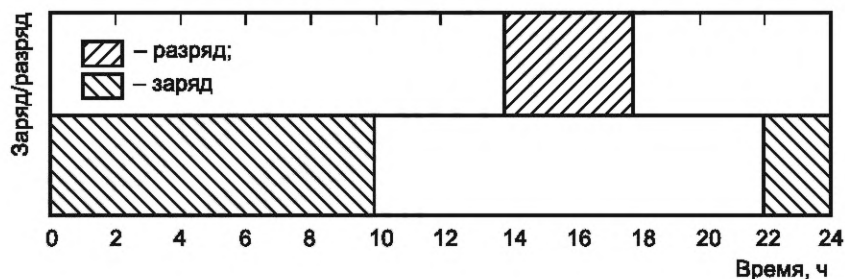
б) Рабочий цикл В срезания пика, период разряда 4 ч
