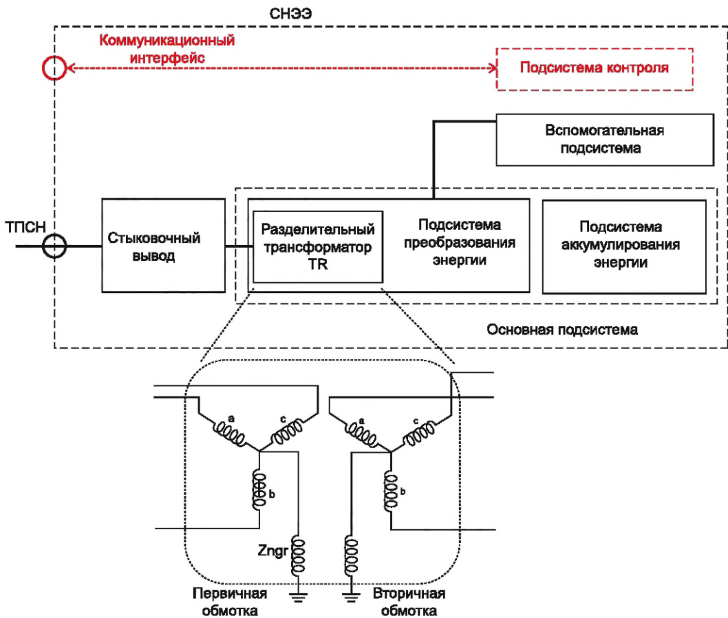
Рисунок А.2 — Соединение электрической сети и СНЭЭ с заземленным Y-заземленным Y (GY-GY)
