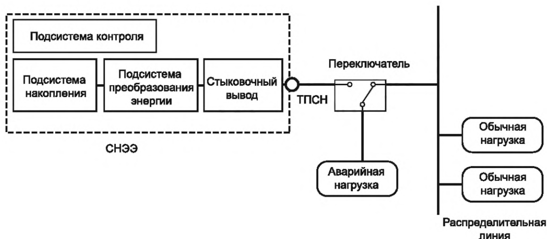
Рисунок 11 — Замена ДГ на СНЭЭ для поддержки резервного электроснабжения
