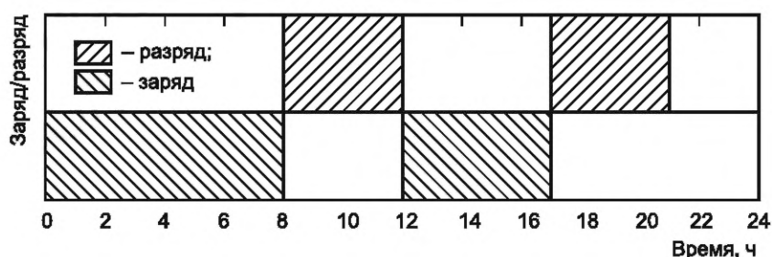
Рисунок 3 — Рабочий цикл «два заряда и два разряда» для срезания пиков
