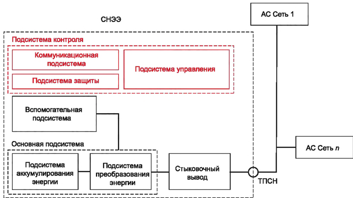
Рисунок А.4 — Нетрансформаторное прямое соединение между электрической сетью и СНЭЭ
