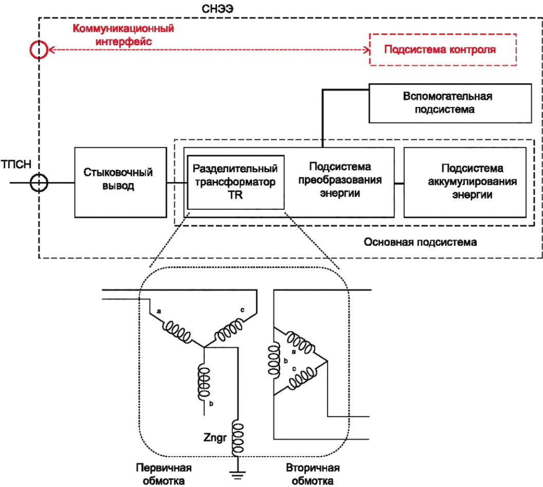
Рисунок А.1 — Соединение электрической сети и СНЭЭ с заземлением Y-Δ (GY-Δ)
