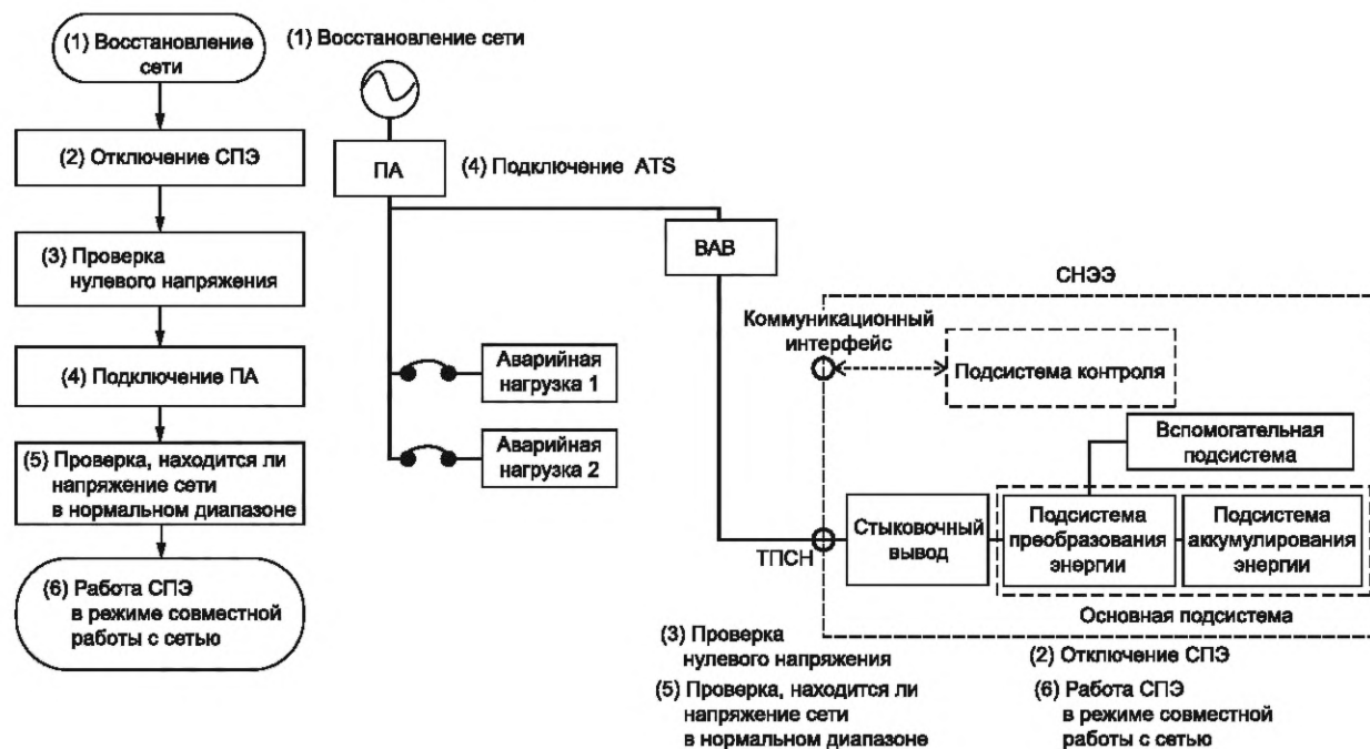
Рисунок 16 — Пример рабочего процесса для поддержки резервного электроснабжения при восстановлении электрической сети
