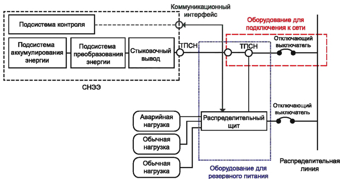
Рисунок 13 — Пример использования СНЭЭ для связи с распределительным щитом
