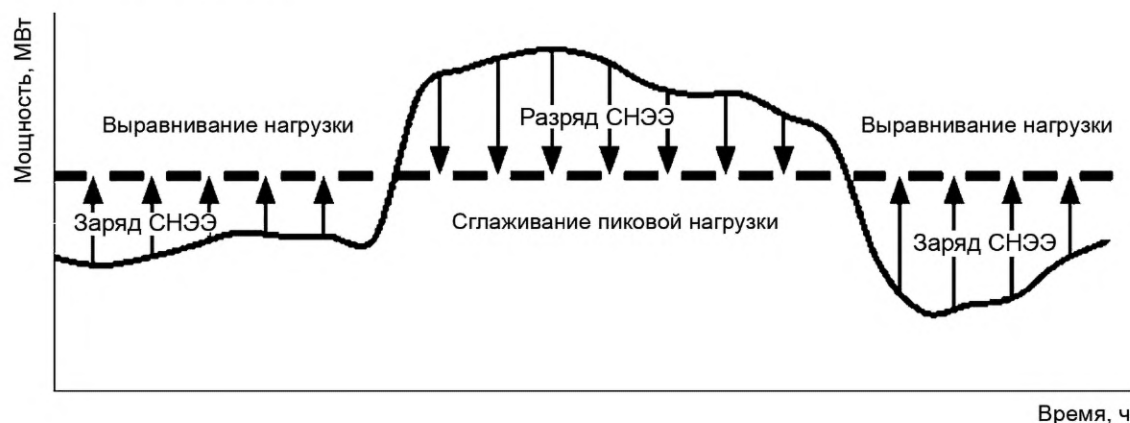
Рисунок 1 — Пример срезания пиков и выравнивания нагрузок потребления с использованием заряда и разряда СНЭЭ
