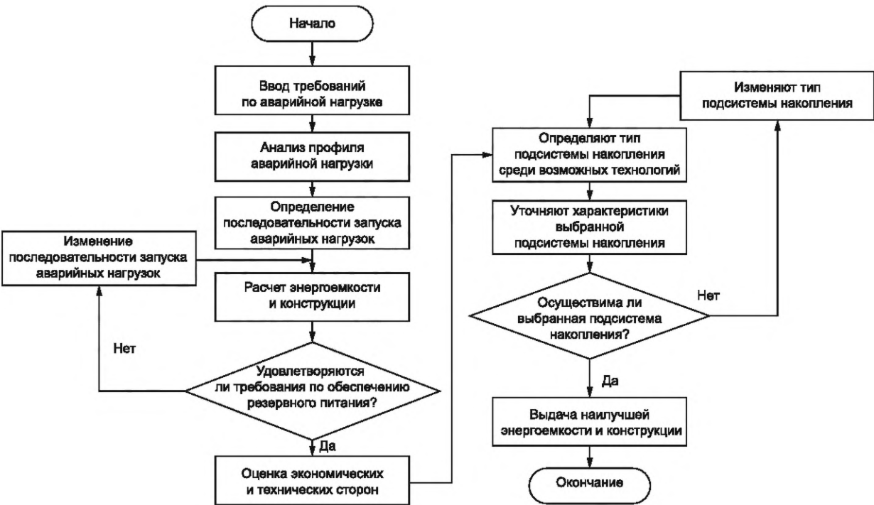
Рисунок 14 — Пример расчета энергетических параметров и проектирования СНЭЭ с функцией резервного электроснабжения и обеспечения питания аварийных нагрузок
