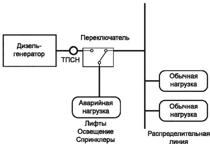
Рисунок 10 — Пример использования резервного электроснабжения с использованием ДГ
