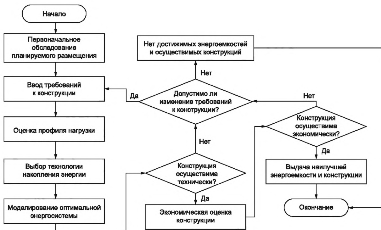
Рисунок 9 — Пример расчета энергетических параметров и проектирования СНЭЭ с функцией работы в ОЭС
