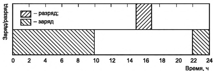
в) Рабочий цикл С срезания пика, период разряда 2 ч
