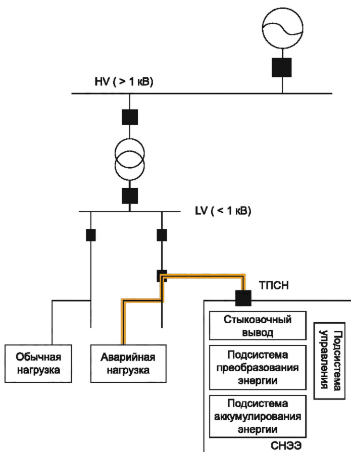
Рисунок 17 — Пример конфигурации для низковольтного присоединения
