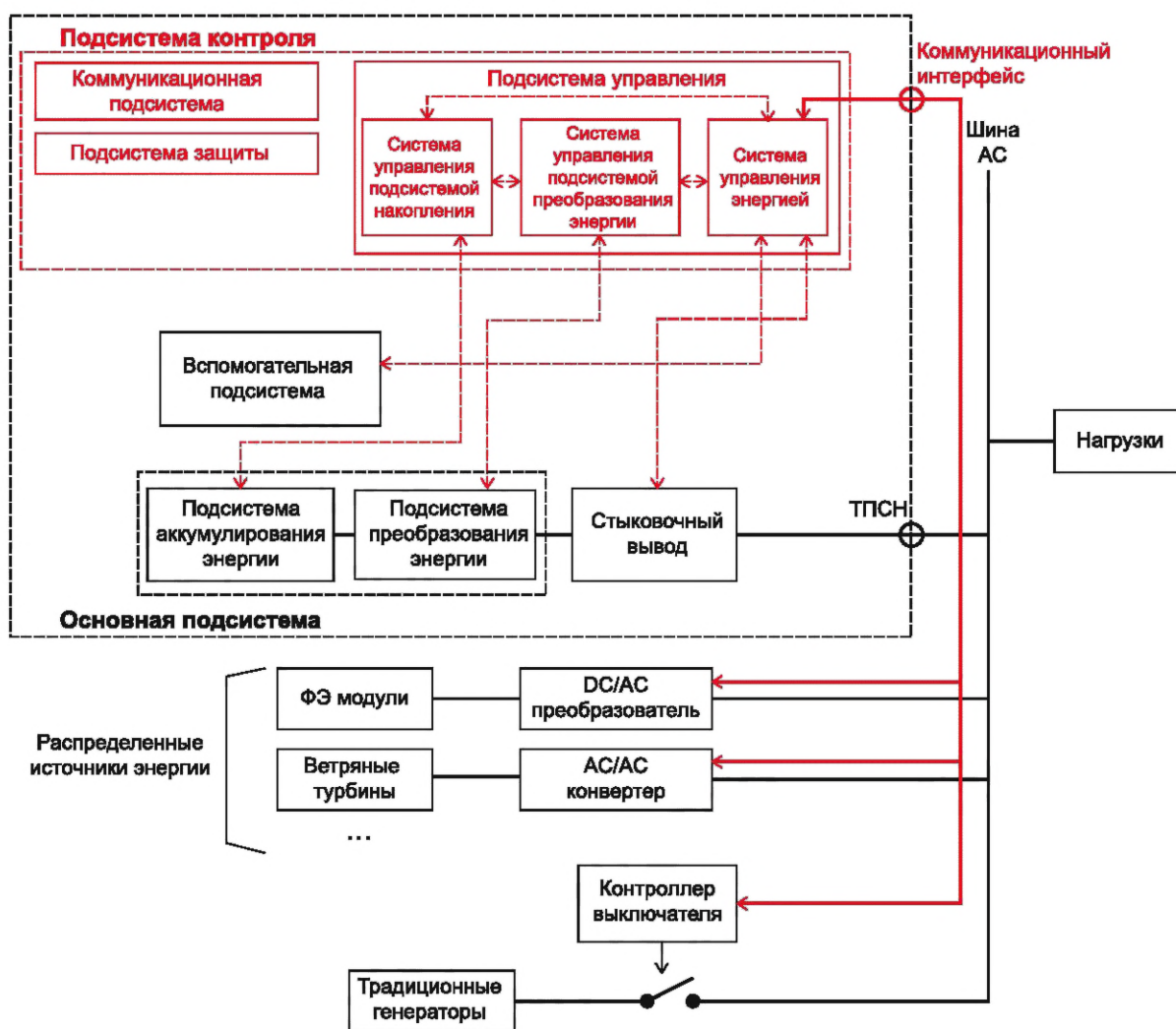
Рисунок 8 — Пример конфигурации при применении СНЭЭ для работы в ОЭС с РИЭ
