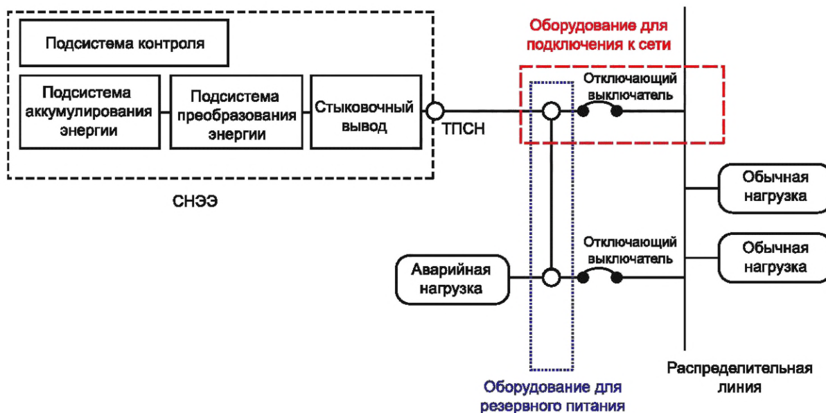
Рисунок 12 — Пример использования СНЭЭ как для резервного электроснабжения, так и для выполнения других функций СНЭЭ
