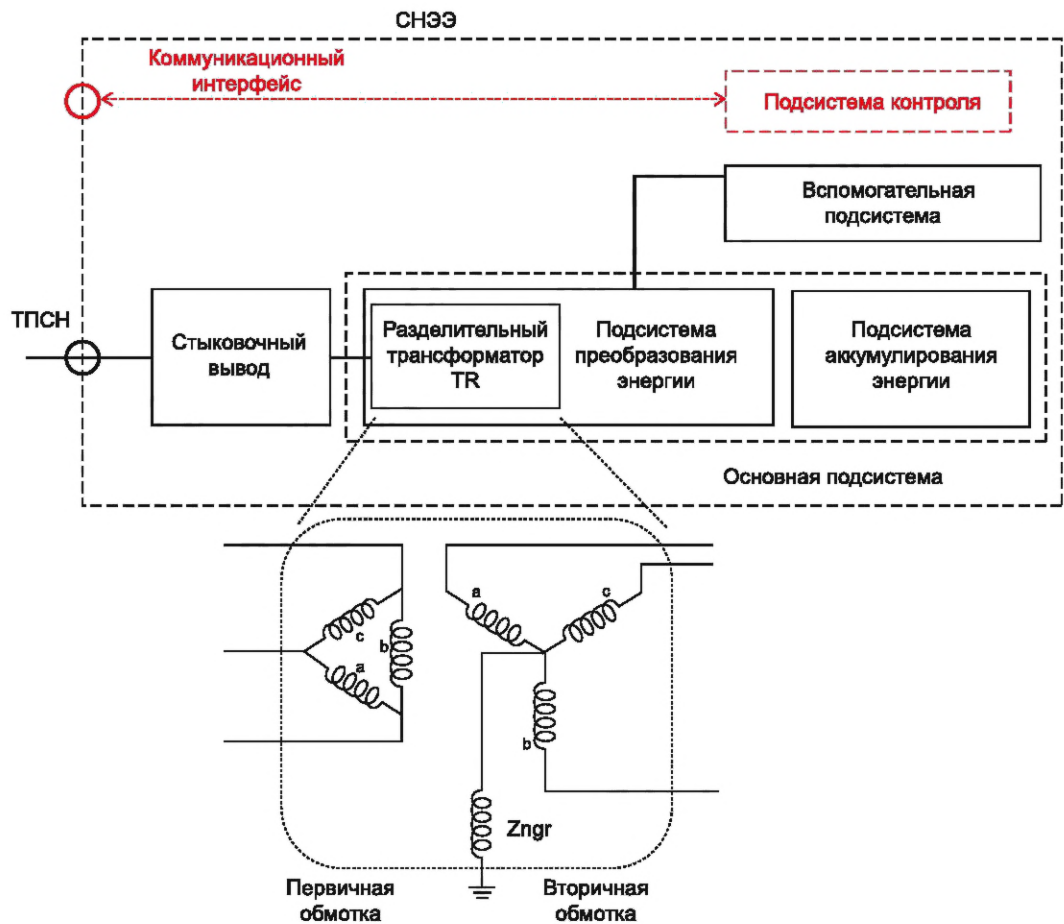
Рисунок А.3 — Соединение электрической сети и СНЭЭ с Δ-заземленным Y (Δ-GY)
