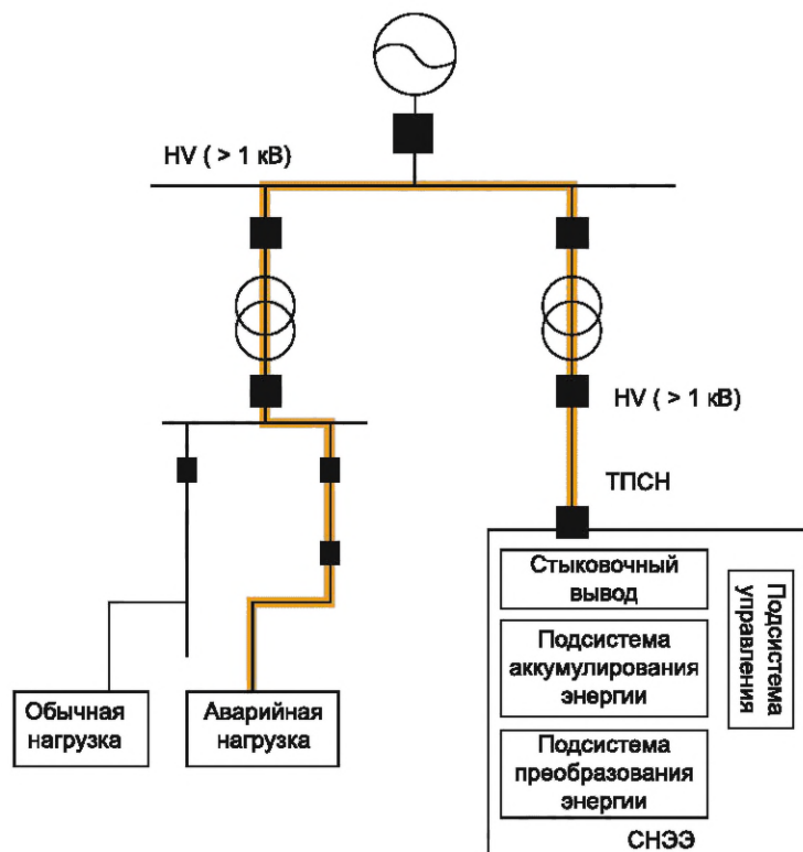
Рисунок 18 — Пример конфигурации для высоковольтного присоединения
