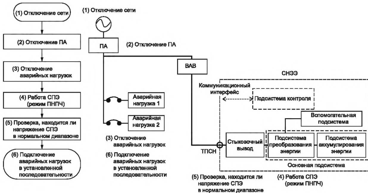
Рисунок 15 — Пример рабочего процесса для поддержки резервного электроснабжения при отключении электрической сети
