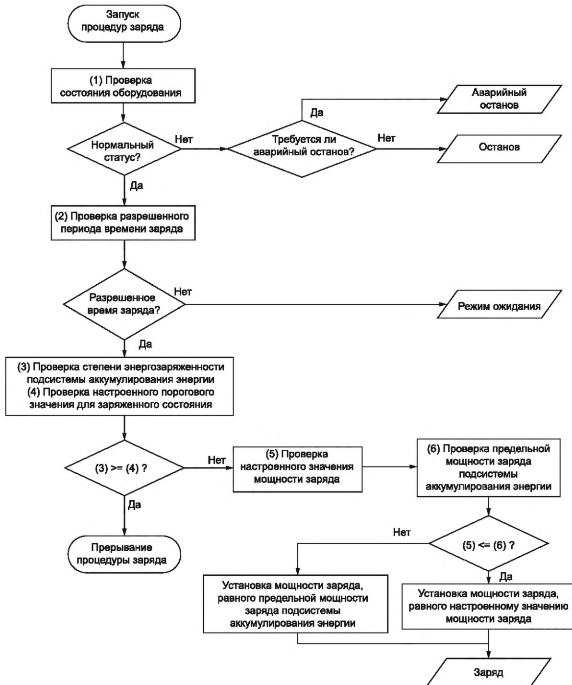
Рисунок 6 — Пример процесса заряда для функции срезания пиков
