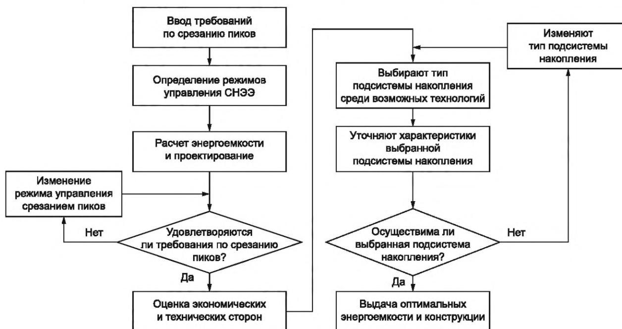
Рисунок 5 — Пример расчета энергетических параметров и проектирования СНЭЭ с функцией срезания пиков и выравнивания нагрузок потребления
