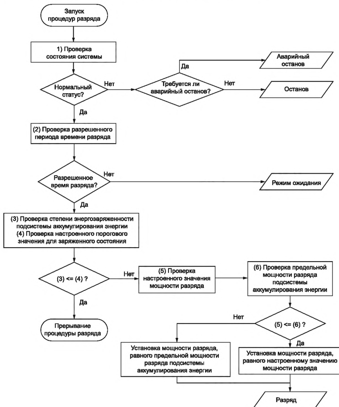
Рисунок 7 — Пример процесса разряда для функции срезания пиков
