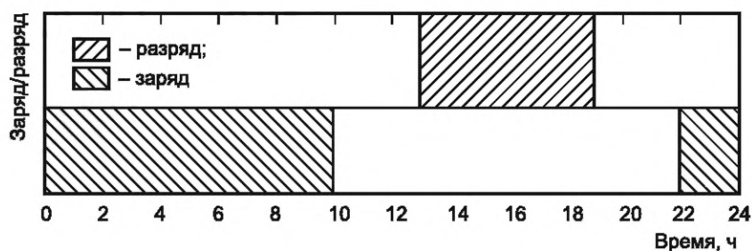
а) Рабочий цикл А срезания пика, период разряда 6 ч
