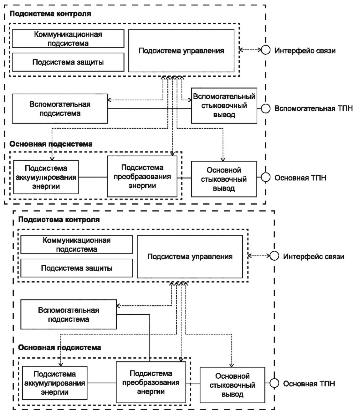
Рисунок 1 — Архитектура СНЭЭ в двух основных конфигурациях СНЭЭ
