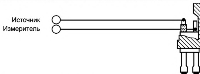
Рисунок 9 — Варианты подключения датчика к измерительному оборудованию
