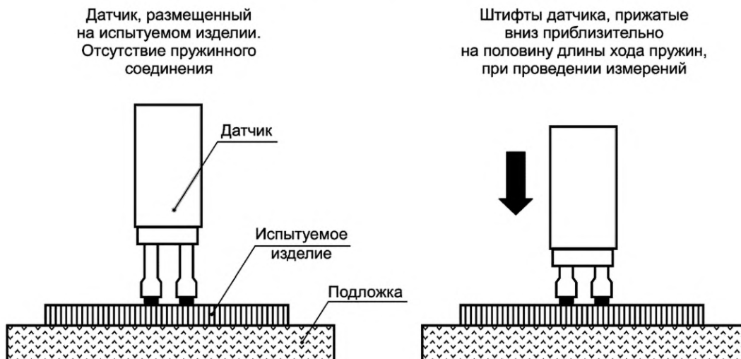
Рисунок 10 — Пример прижатия пружин при проведении испытаний
