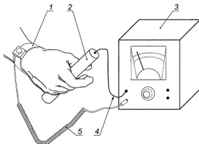
3а — Испытания с использованием омметра
