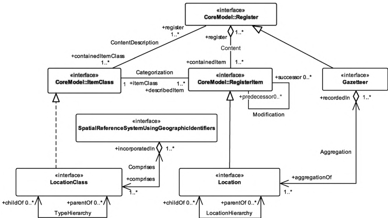
Рисунок 1 — Обзор концептуальной схемы
