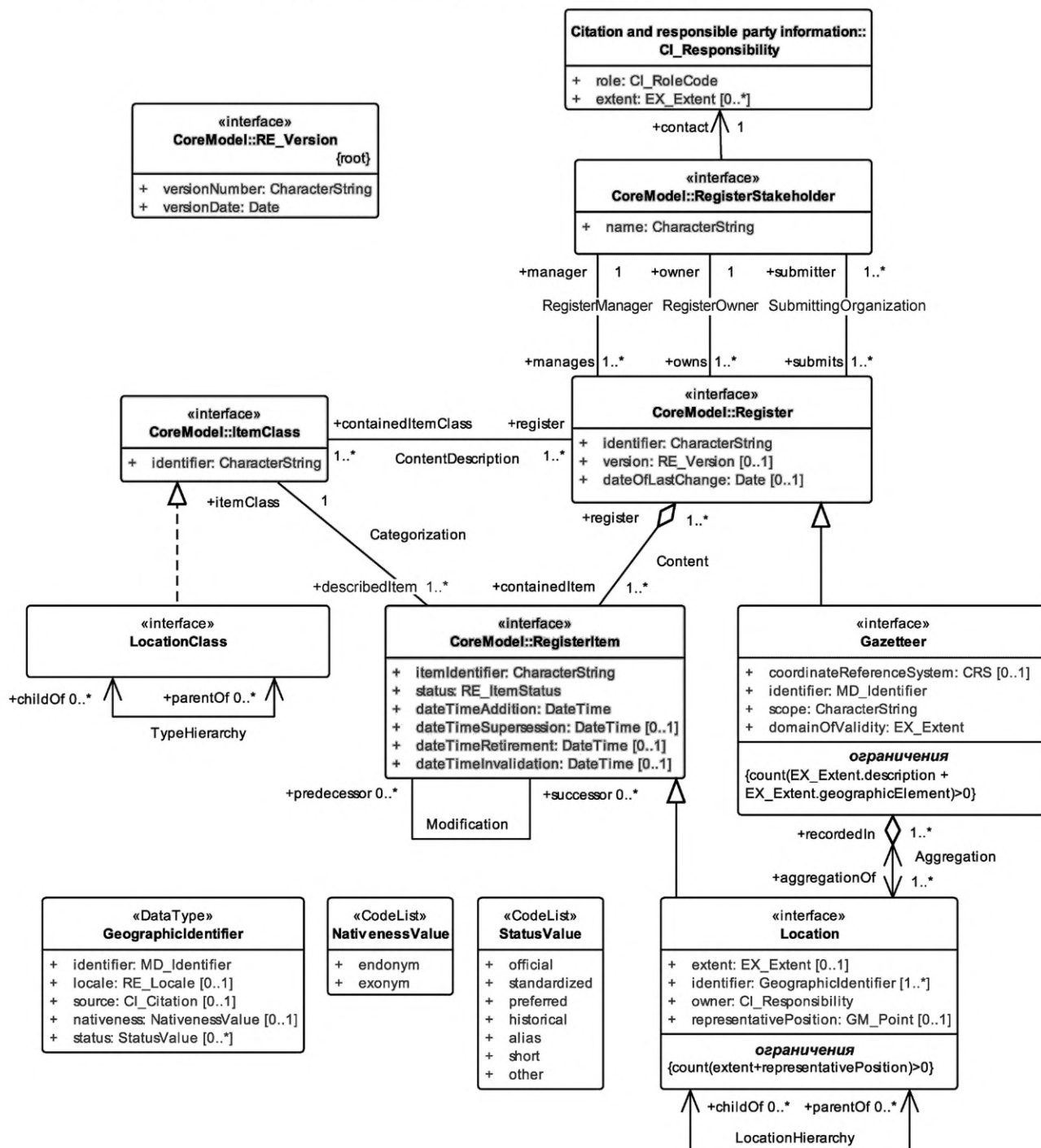
Рисунок 3 — Концептуальная схема. Географический справочник
