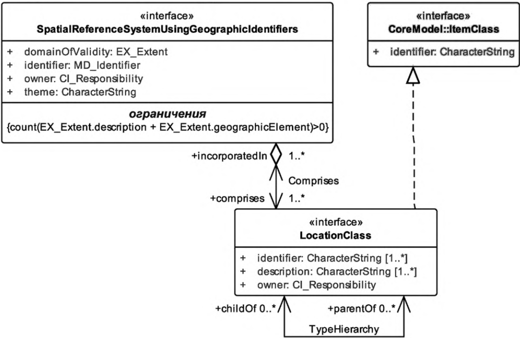
Рисунок 2 — Концептуальная схема. Пространственная привязка с использованием географических идентификаторов
