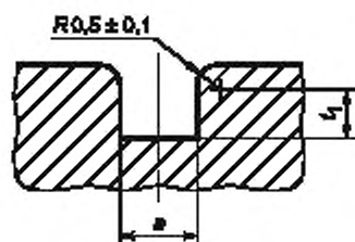
Рисунок А.1 — Шлиц испытательного оборудования для типа 6 исполнения А рабочей части отвертки
