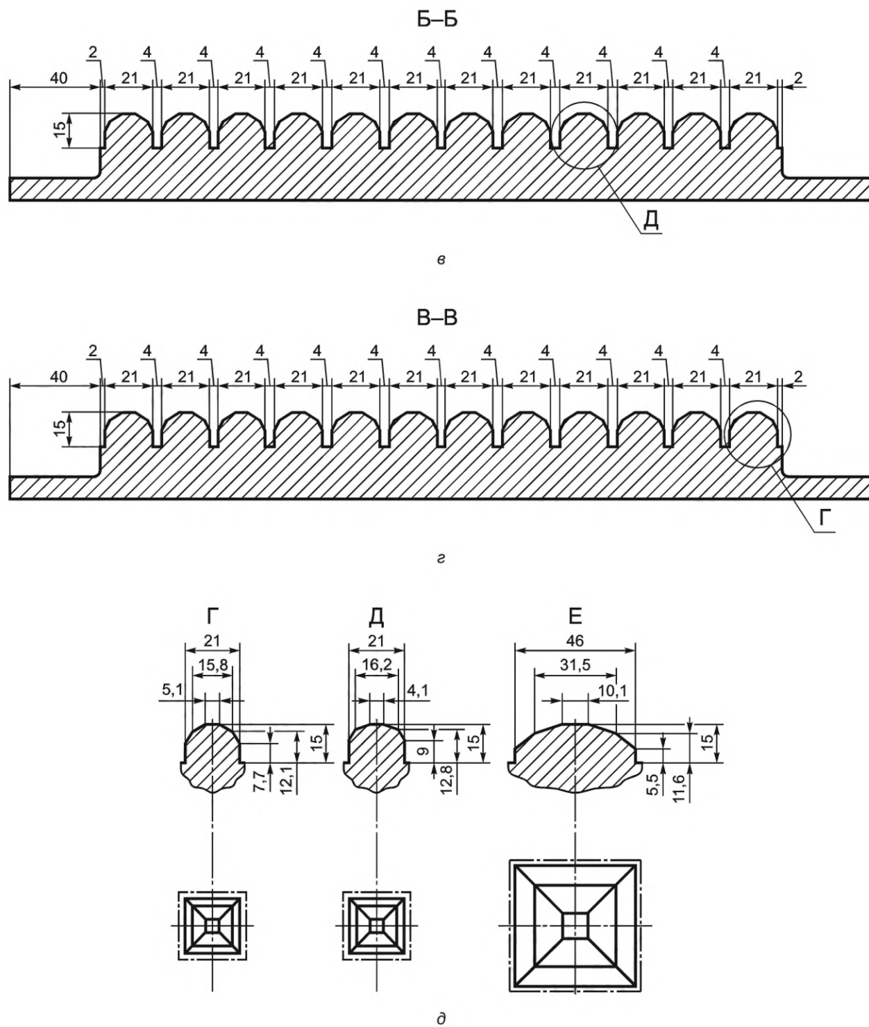
Рисунок А.1 — Геометрические размеры щебеночной плиты
