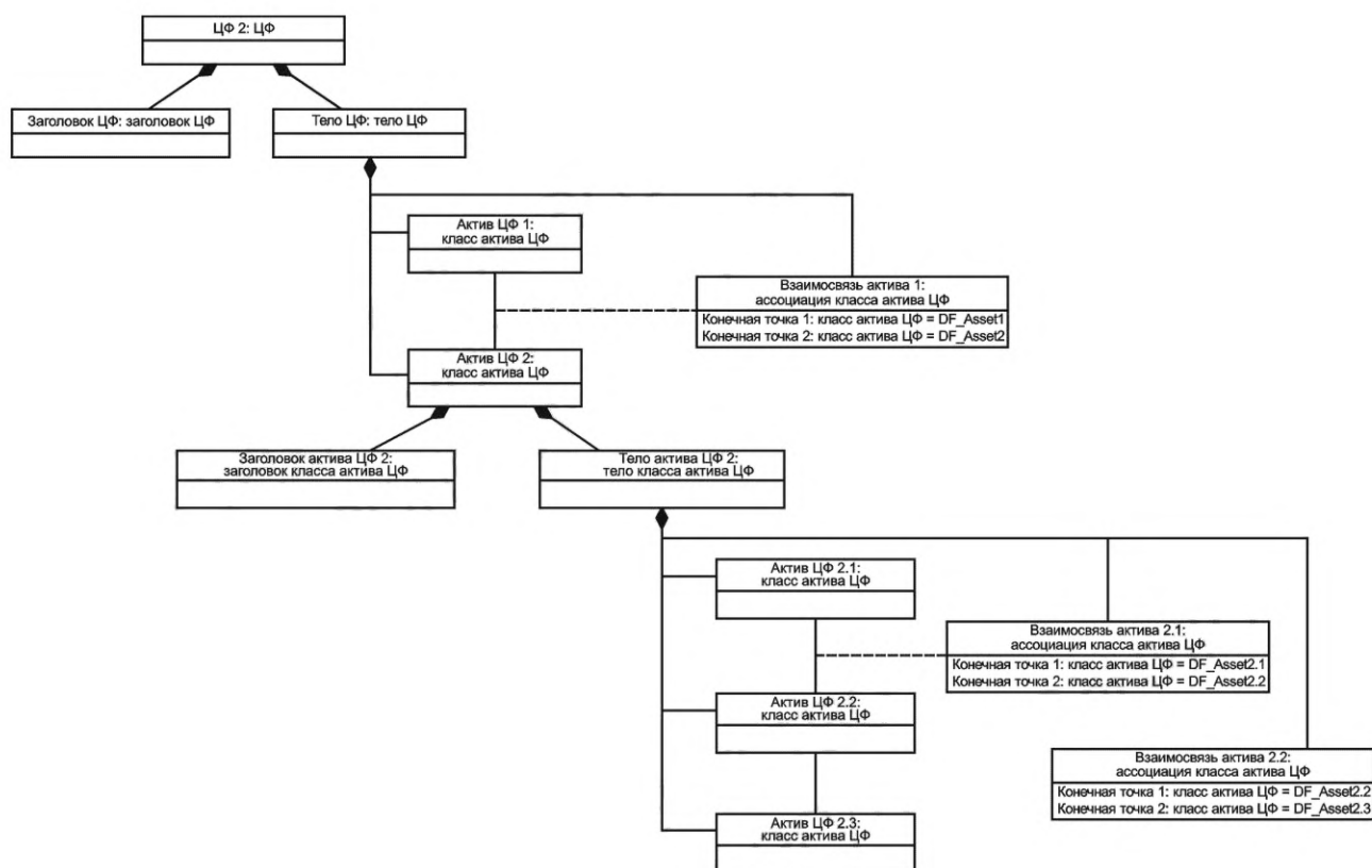
Рисунок А.10 — Цифровая фабрика, имеющая составные активы
